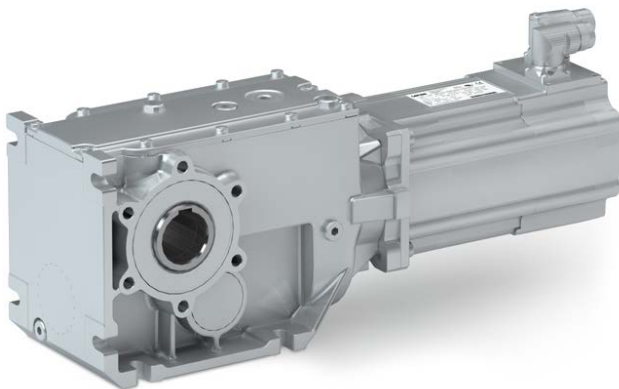
Servo-Synchronmotor MCS12L - Kegelradgetriebe g500-B450
