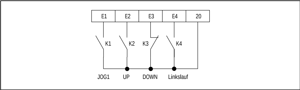
FIG 7-4 Ansteuerung der Motorpotentiometerfunktion, C007= -22-
