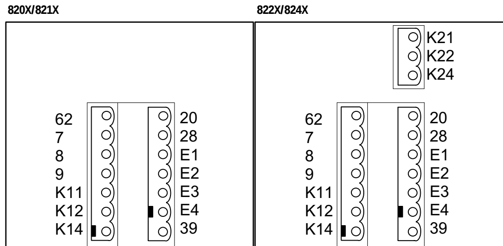
FIG 4-23 Lage der Steuerklemmen
