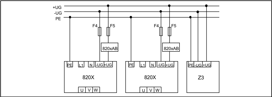
FIG 10-2 Prinzipschaltbild: Zentrale Einspeisung bei Verbundbetrieb 820X F4, F5 Sicherungen auf der DC-Ebene, s. Zubehör Z3 Bremsschopper/Bremsmodul, s. Zubehör 820XAB Strombegrenzungsbaugruppe, s. Zubehör
