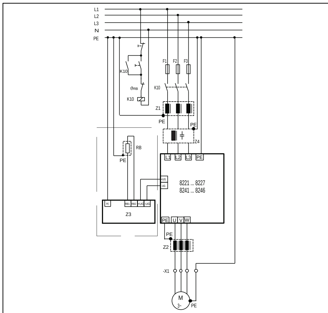
FIG 4-22 Leistungsanschlüsse 822X/824X
