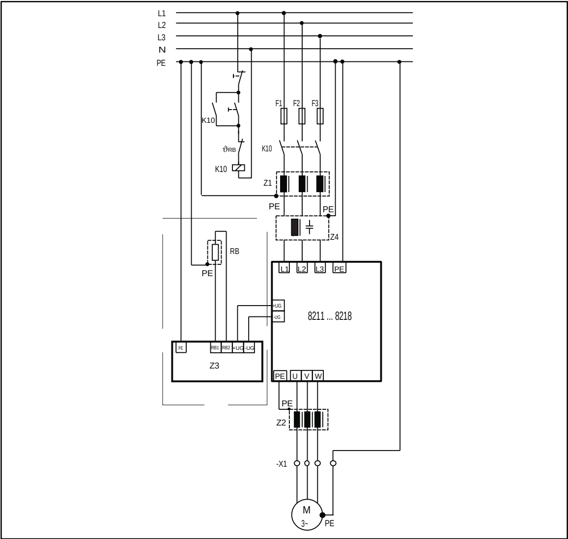
FIG 4-21 Leistungsanschlüsse 821X
