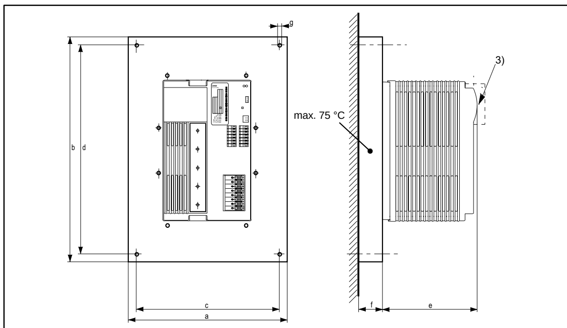
FIG 4-12 Abmessungen 821X-V003: Wandmontage mit Lenze-Konvektionskühler
