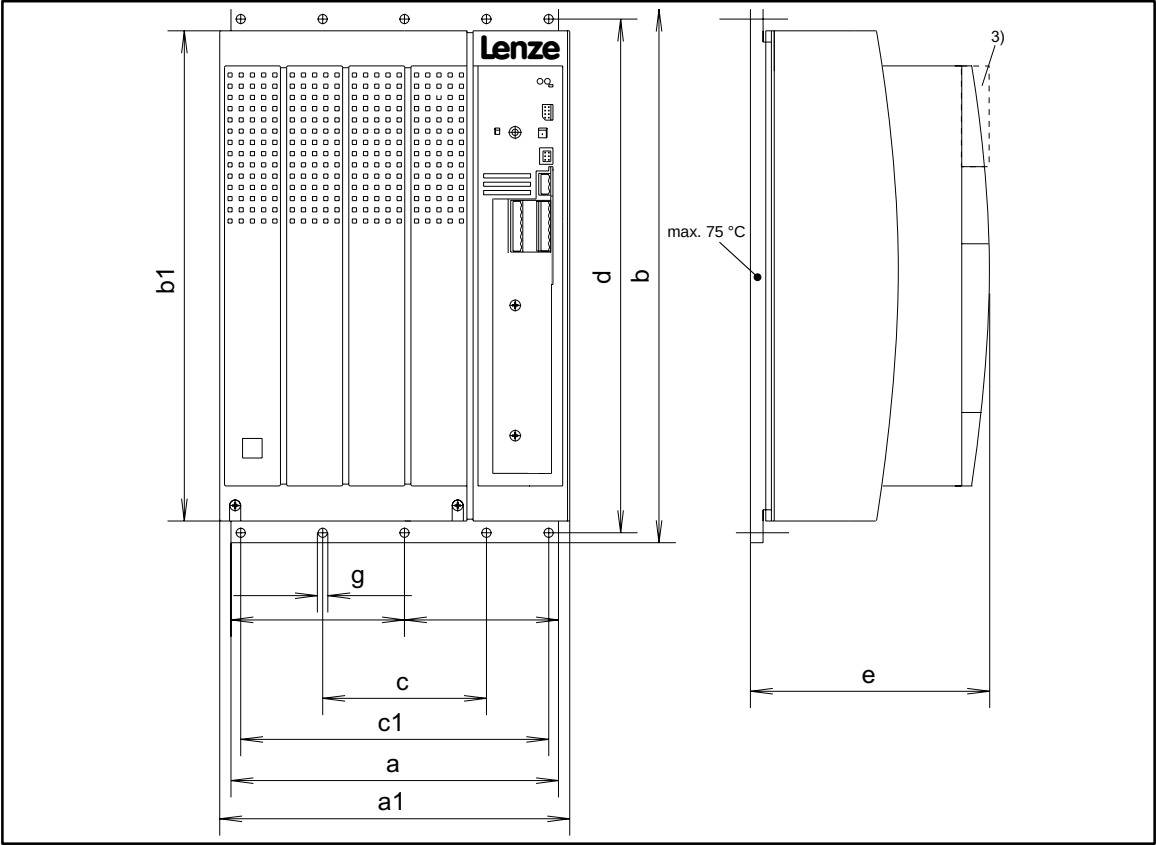
FIG 4-13 Abmessungen 822X-C-V003: Montage im Schaltschrank
