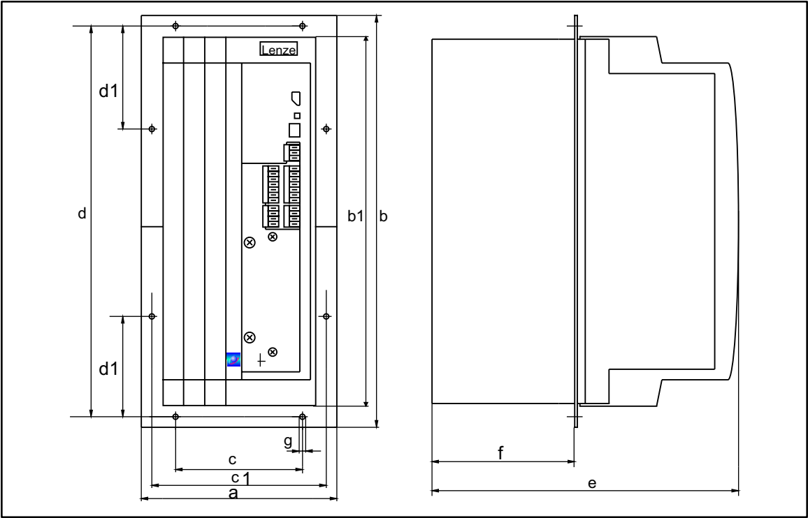
FIG 4-10 Abmessungen 8241 - 8246: Montage mit thermisch separiertem Leistungsteil
