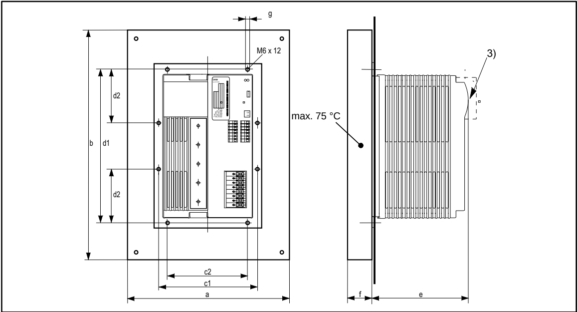
FIG 4-11 Abmessungen 821X-V003: Montage im Schaltschrank mit Lenze-Konvektionskühler
