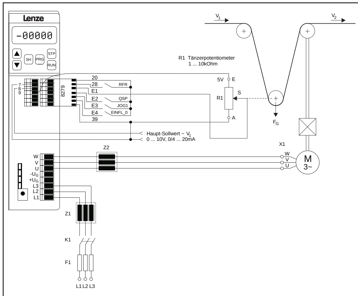
FIG 15-3 Einsatz einer Tänzerlageregelung
