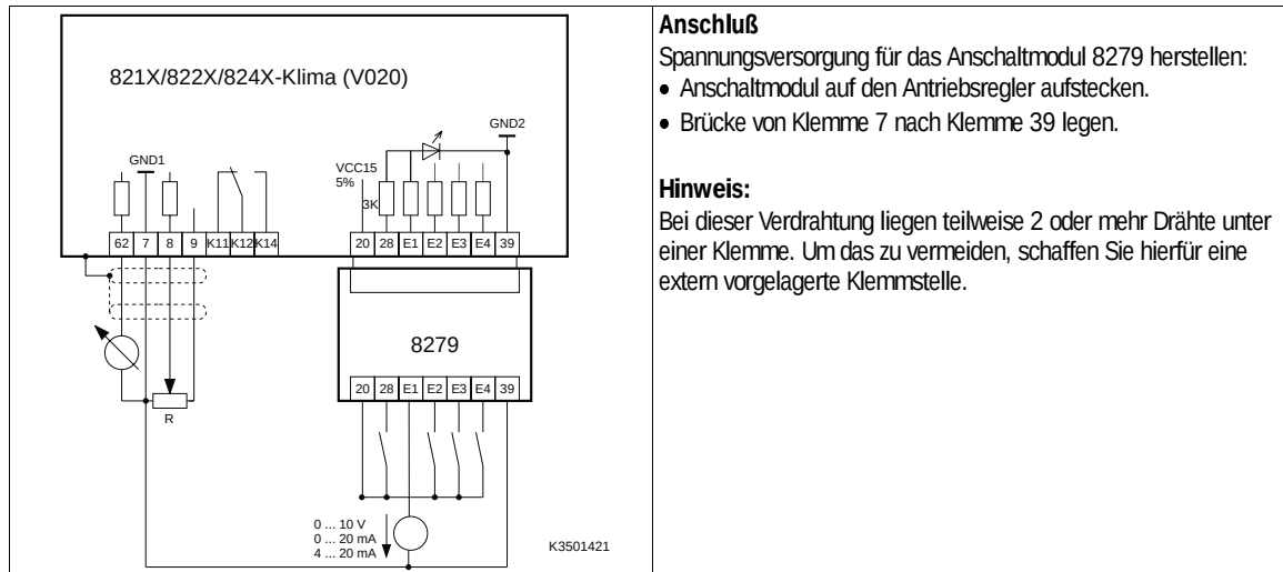
FIG 4-26 Steueranschlüsse: Versorgung mit interner Steuerspannung
