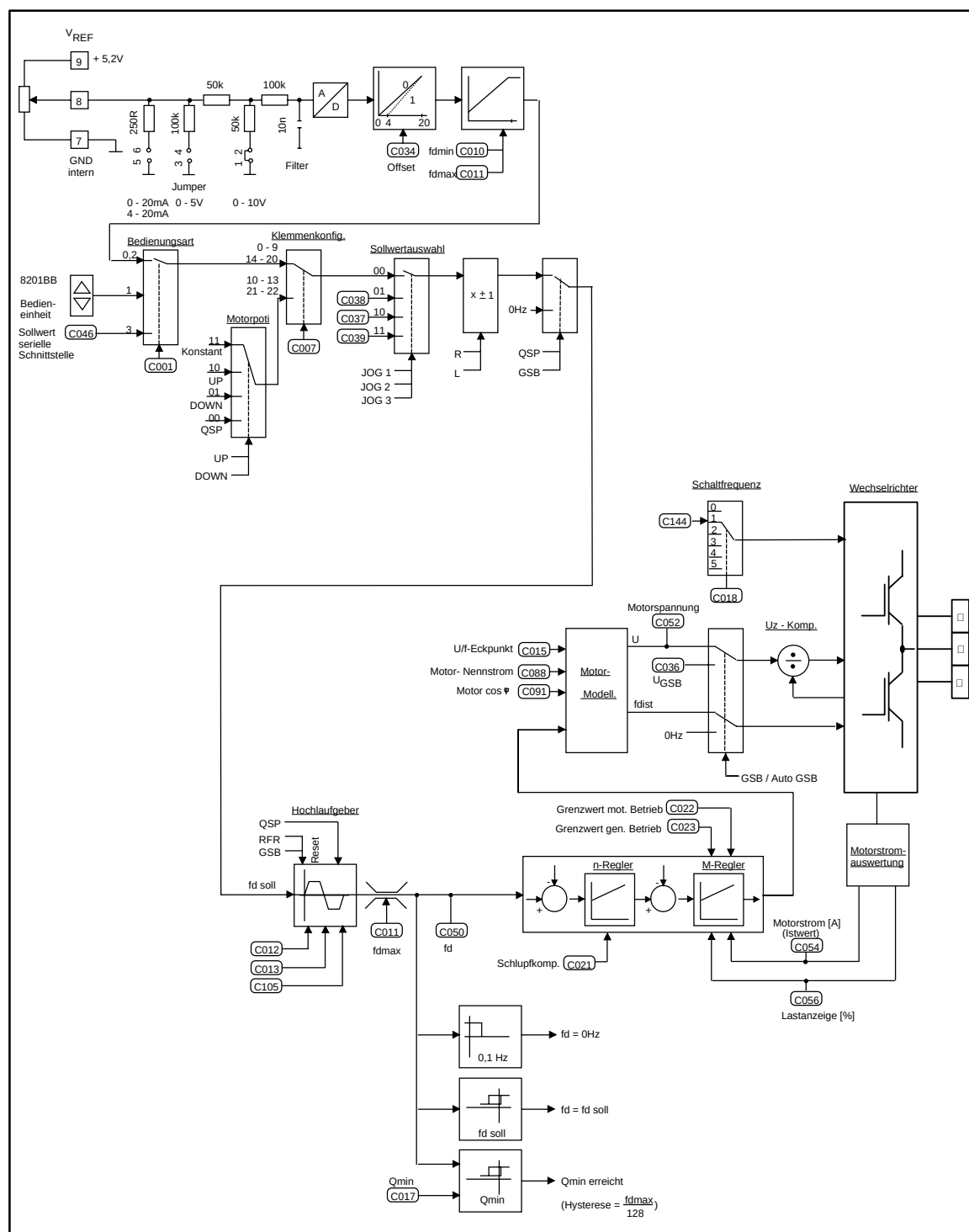
FIG 16-5 Signalfuß 821X/822X/824X: Regelstruktur Betriebsart Motorstrom-Regelung
