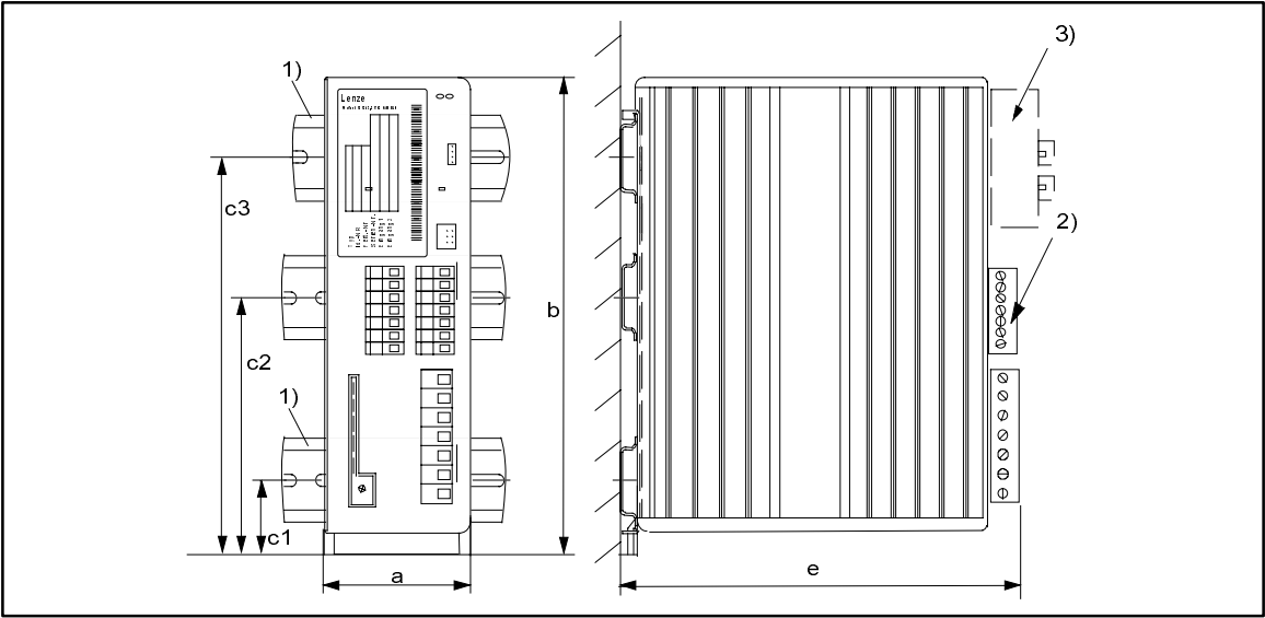
FIG 4-7 Abmessungen 8211 - 8214: Montage auf Hutschienen
