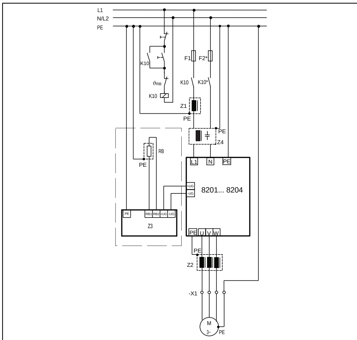
FIG 4-20 Leistungsanschlüsse 820X
