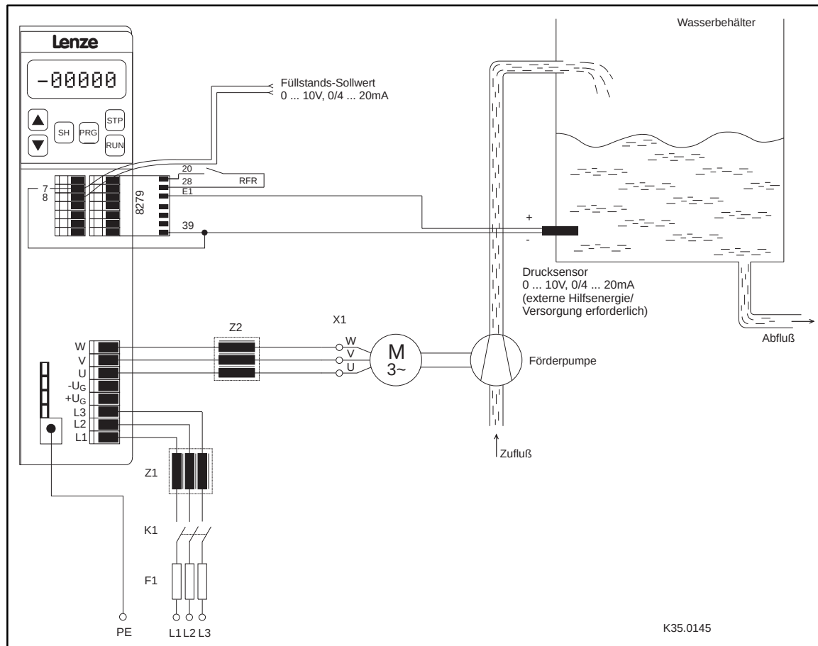
FIG 5-3 Einsatz einer Pumpe mit Niveauregelung
