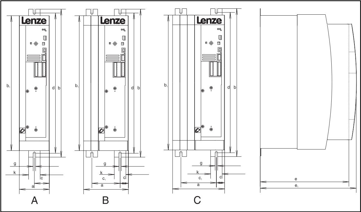
FIG 4-5 Abmessungen 8241 - 8246: Standardmontage
