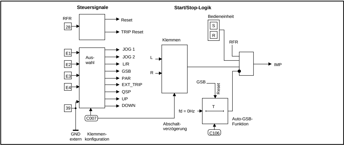
FIG 16-2 Signalfluß 820X: Steuerung der Antriebsregler
