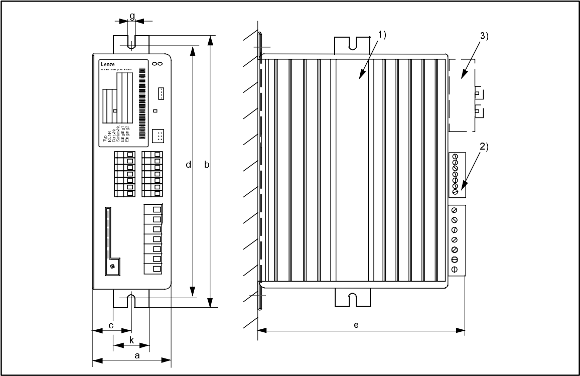
FIG 4-1 Abmessungen 8201 - 8204: Standardmontage
