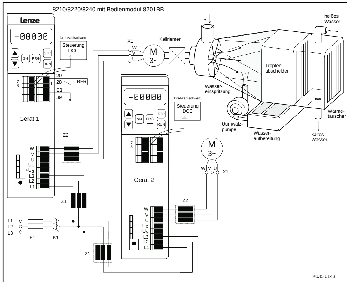
FIG 15-4 Anwendungsbeispiel einer Klimaanlage
