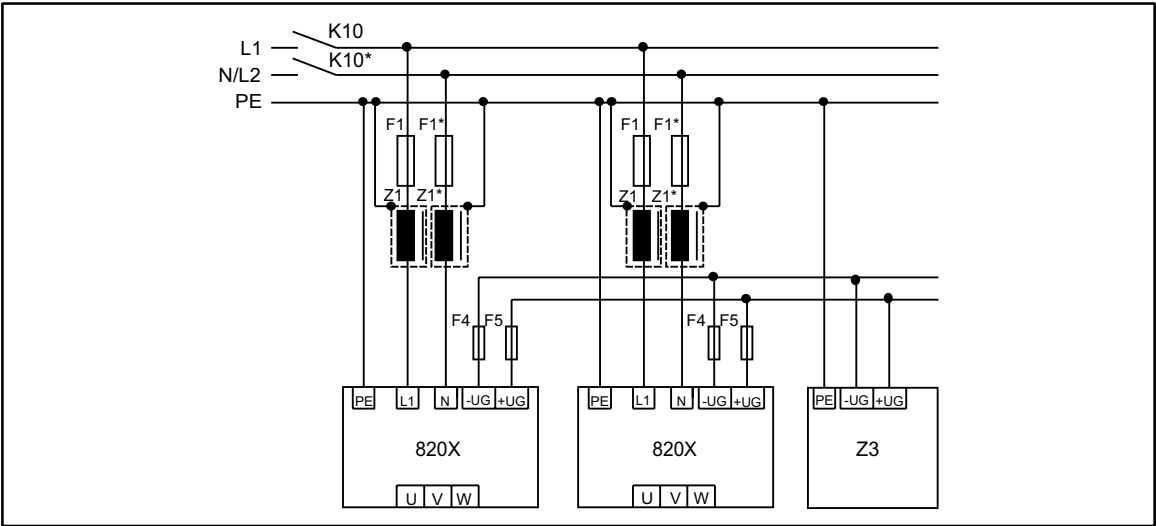
FIG 10-4 Prinzipschaltbild: Dezentrale Einspeisung bei Verbundbetrieb 820X
