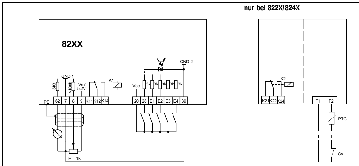
FIG 4-24 Steueranschlüsse: Versorgung mit interner Steuerspannung
