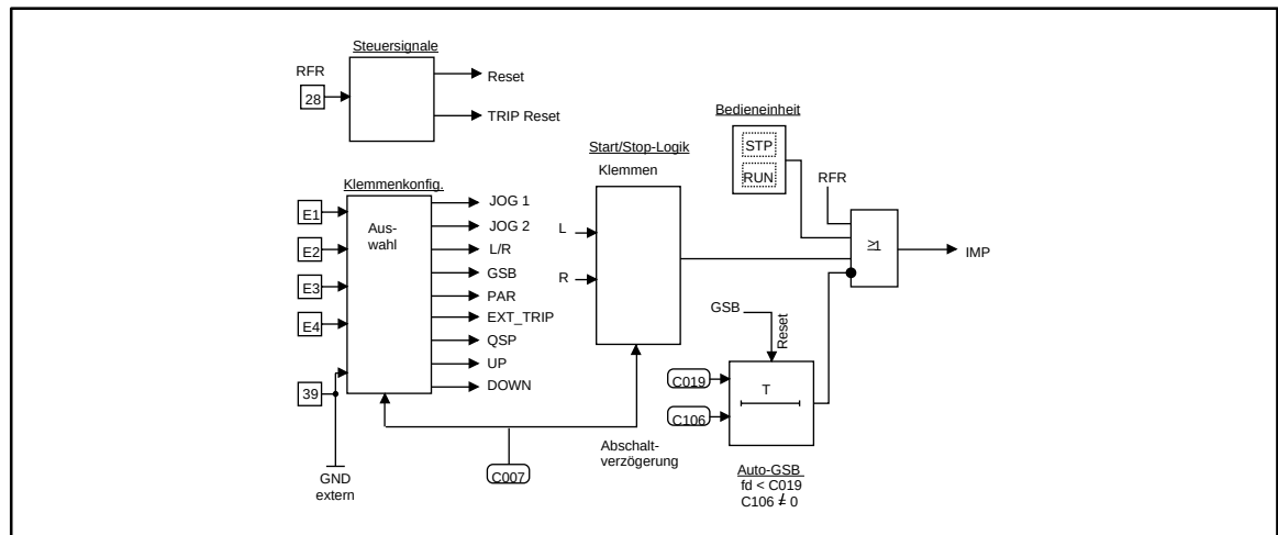
FIG 16-6 Signalfluß 821X/822X/824X: Steuerung der Antriebsregler
