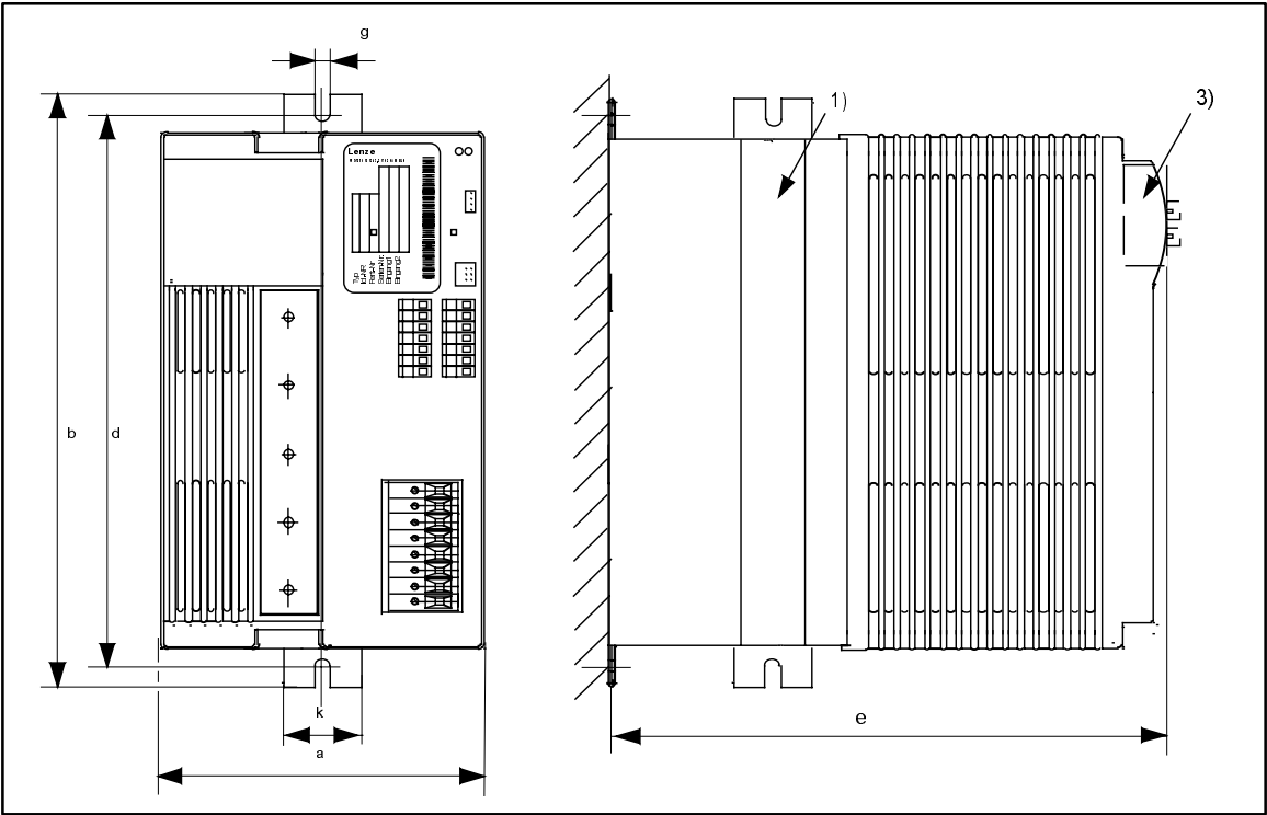
FIG 4-3 Abmessungen 8215 - 8218: Standardmontage
