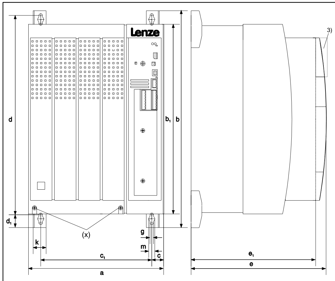
FIG 4-4 Abmessungen 8221 - 8227: Standardmontage
