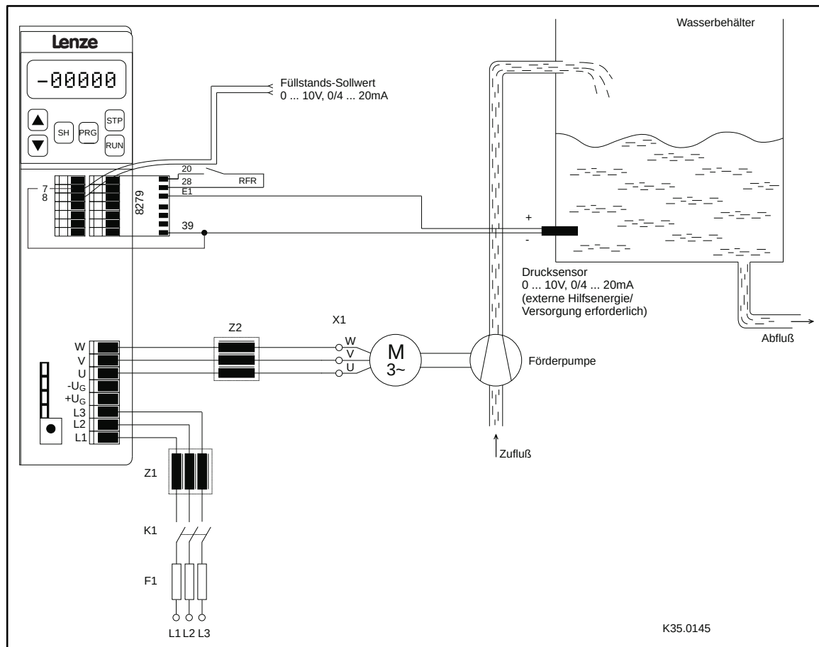
FIG 15-2 Einsatz einer Pumpe mit Niveauregelung
