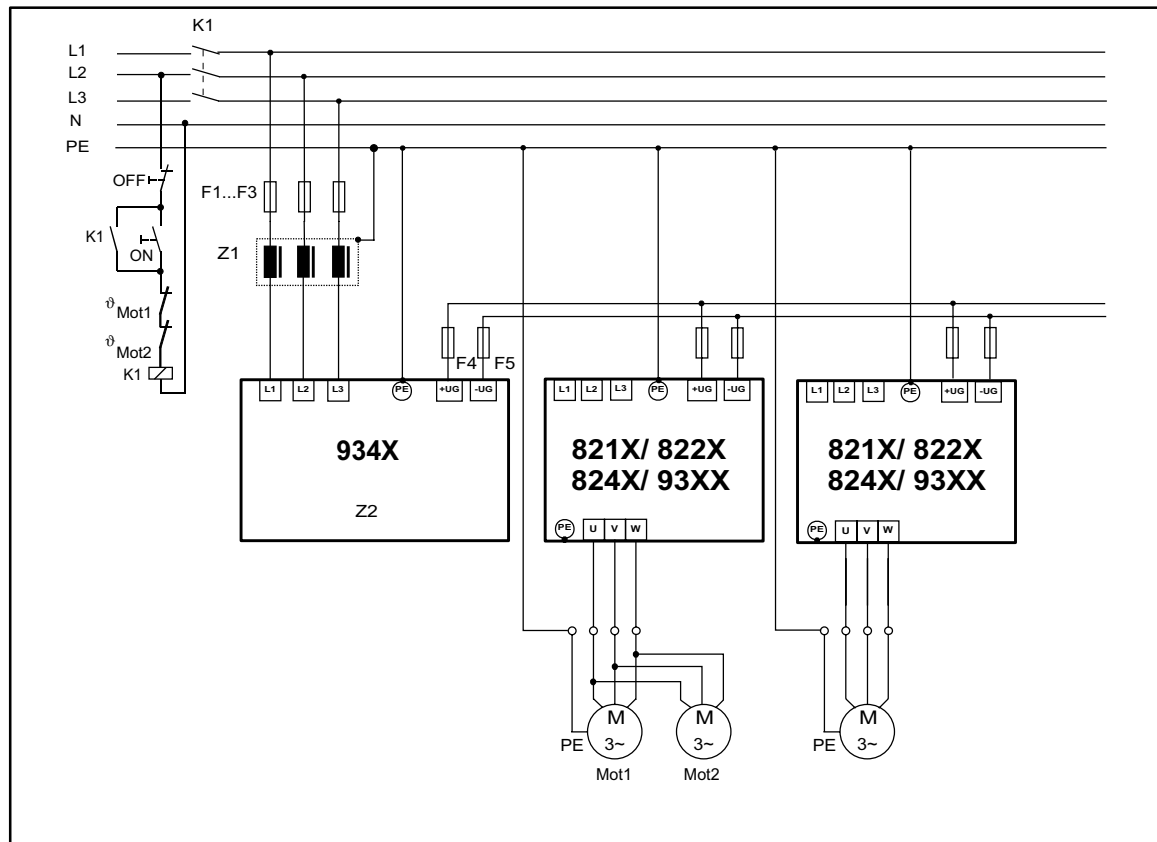
FIG 10-3 Prinzipschaltbild: Zentrale Einspeisung bei Verbundbetrieb 821X/822X/824X/93XX Z1 Netzfilter/-drossel Z2 Versorgungs- und Rückspeisemodul F1 ... F5 Absicherung K1 Hauptschütz
