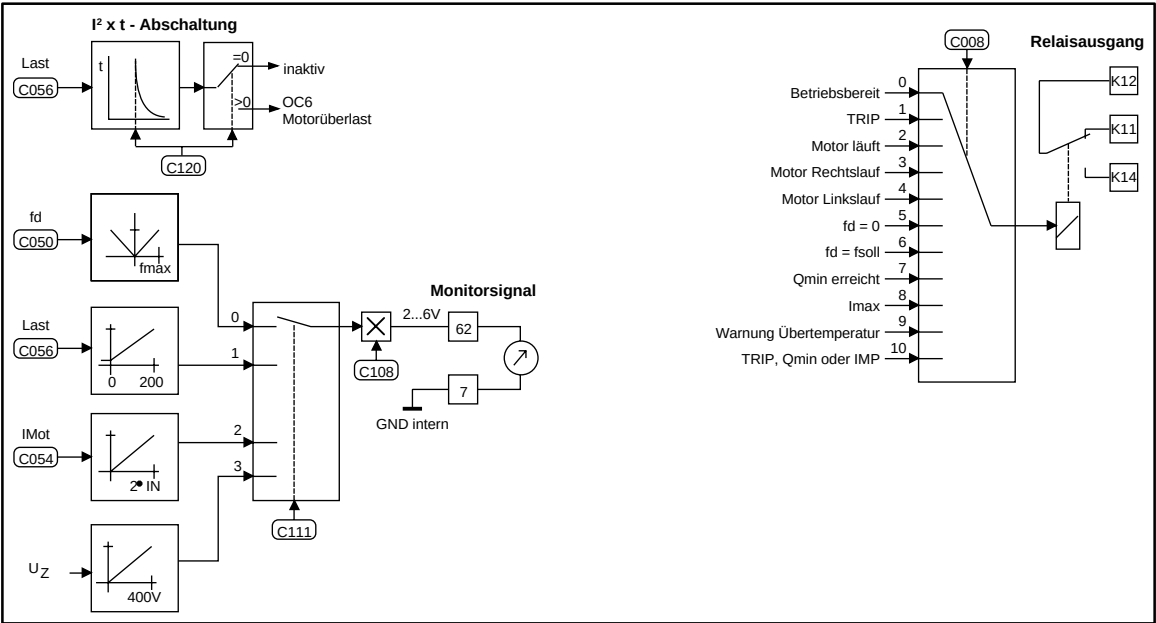
FIG 16-3 Signalfluß 820X: Überwachungen
