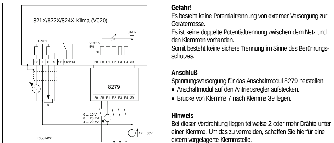
FIG 4-27 Steueranschlüsse: Versorgung mit externer Steuerspannung (+12 V ... +30 V)
