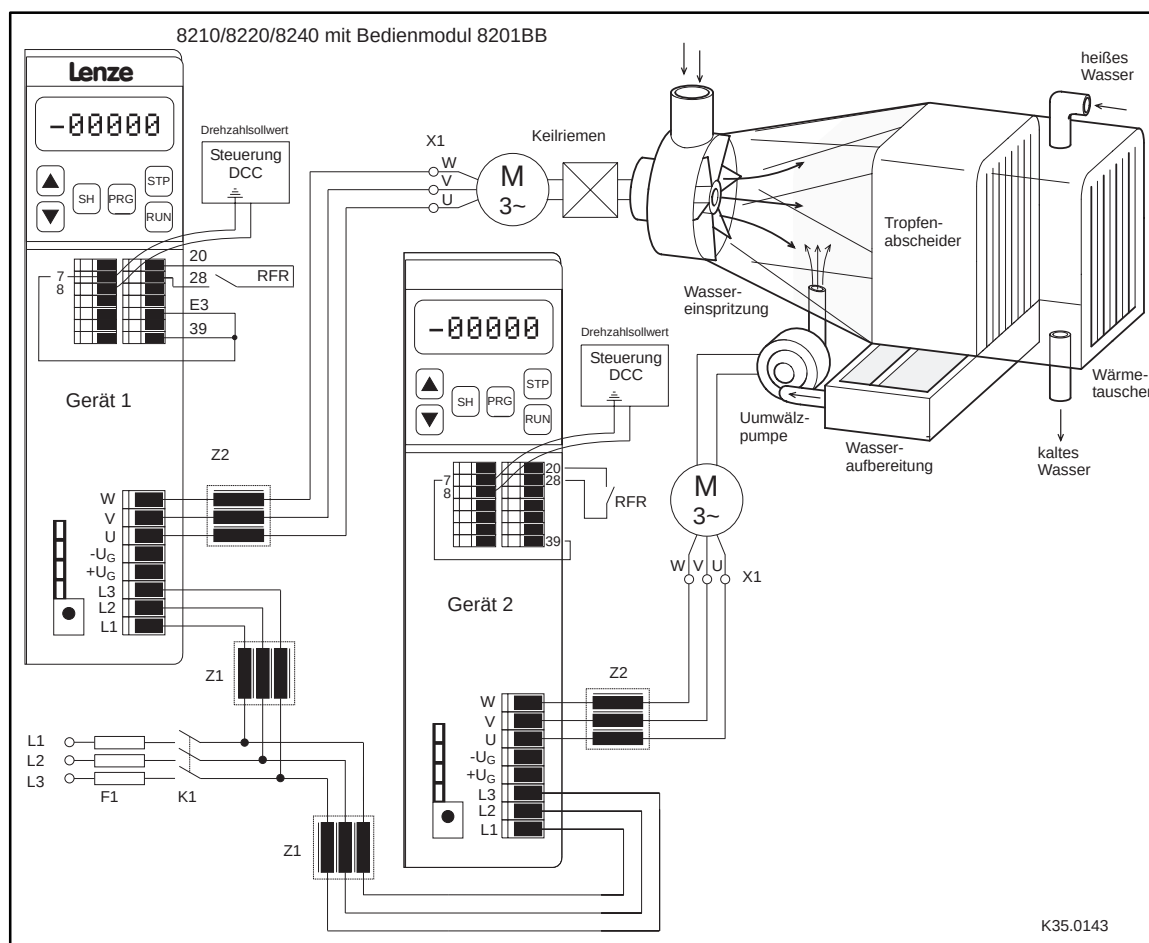
FIG 5-5 Anwendungsbeispiel einer Klimaanlage
