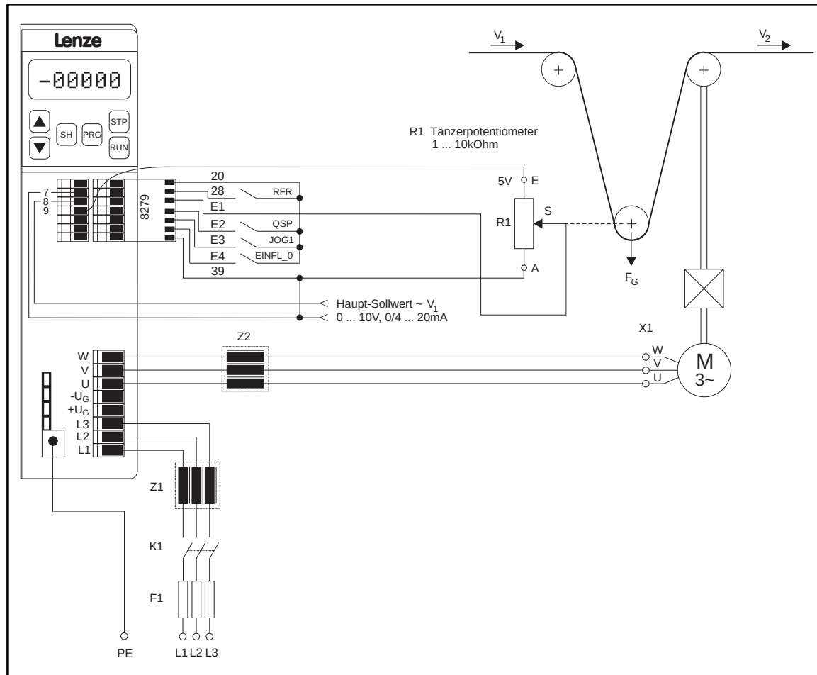
FIG 5-4 Einsatz einer Tänzerlageregelung
