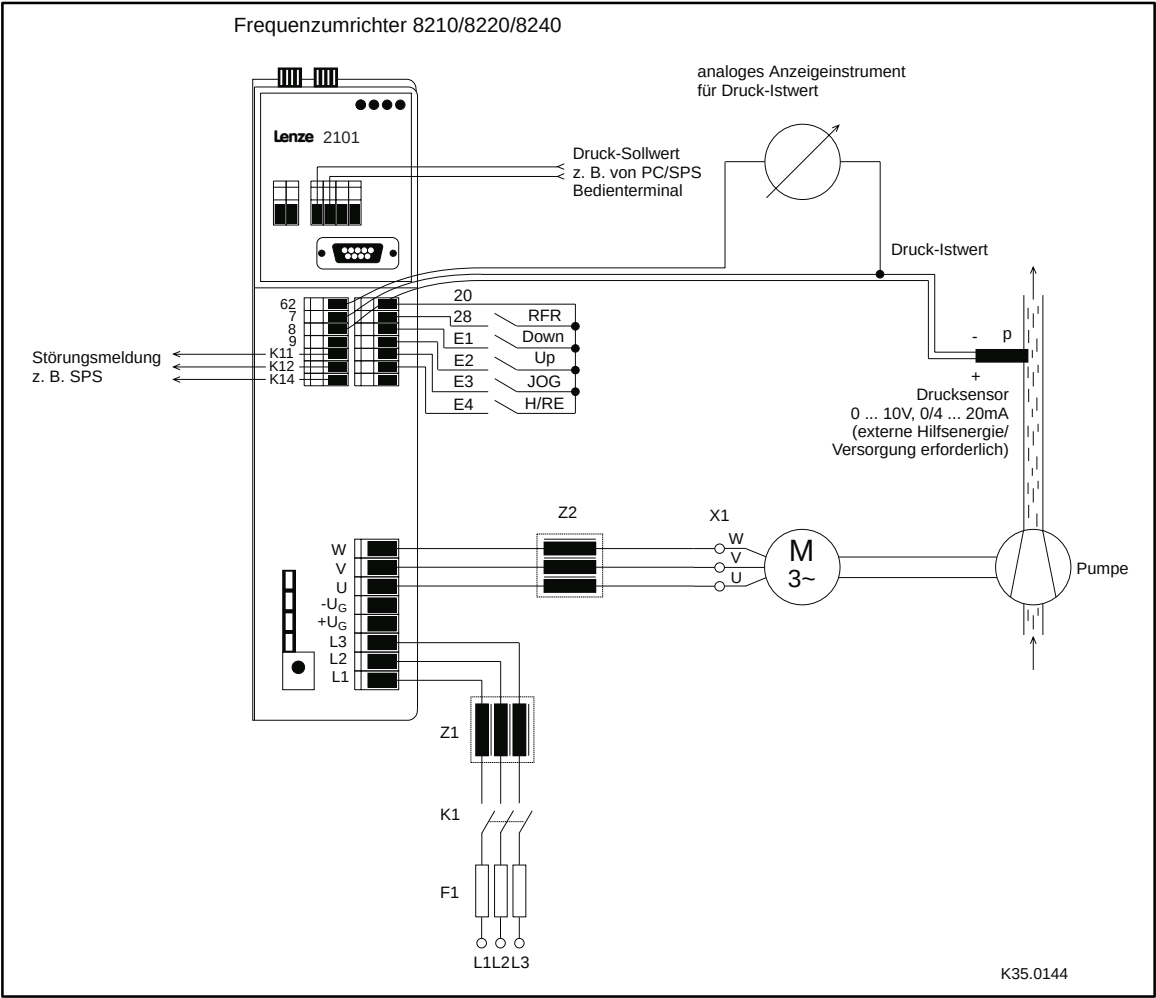
FIG 15-1 Einsatz einer Pumpe mit Druckregelung
