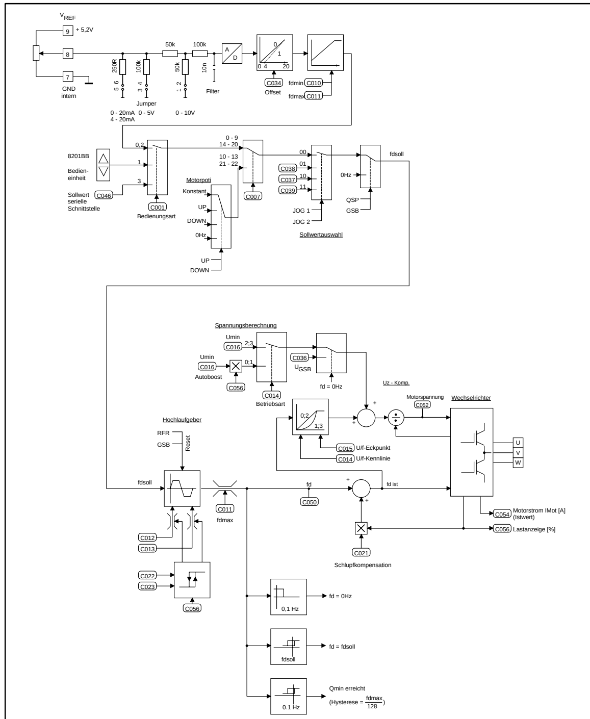
FIG 16-1 Signalfluß 8200: Regelstruktur
