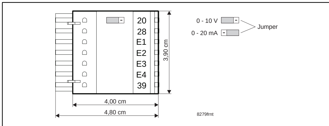
FIG 3-2 Abmessungen Analoges Anschaltmodul
