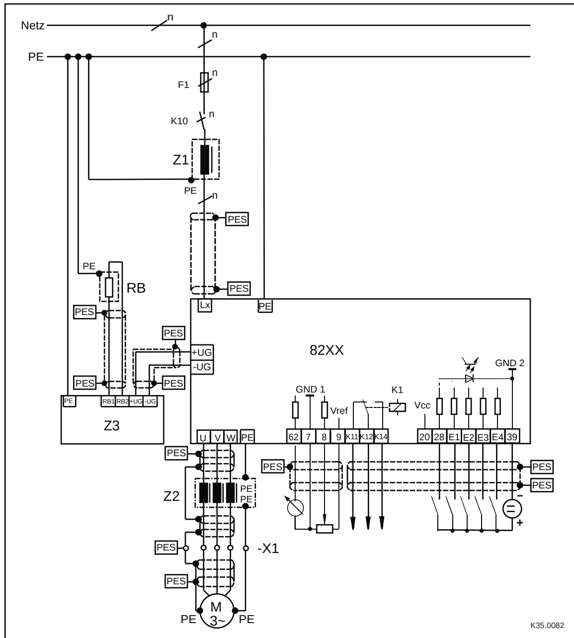
FIG 4-28 Beispiel für eine EMV-gerechte Verdrahtung
