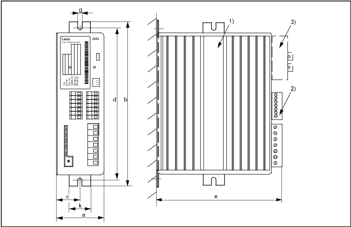
FIG 4-2 Abmessungen 8211 - 8214: Standardmontage
