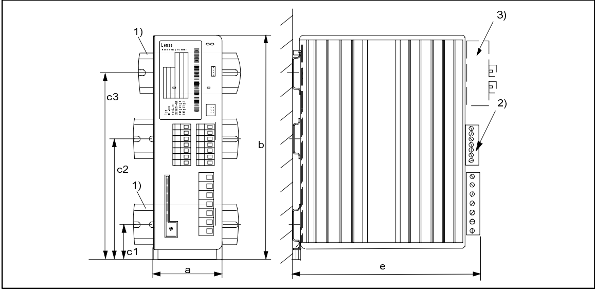
FIG 4-6 Abmessungen 8201 - 8204: Montage auf Hutschienen
