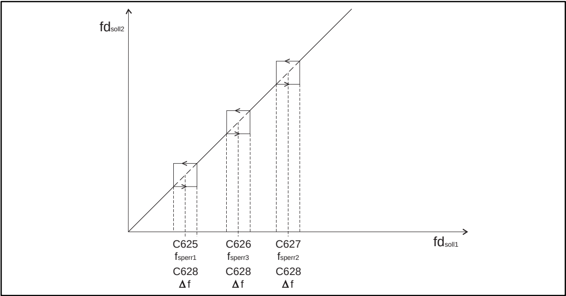
FIG 7-3 Sperrfrequenzen und ihre Bandbreite ( \Delta f )
