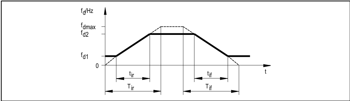
FIG 5-1 Hoch- und Ablaufzeiten
