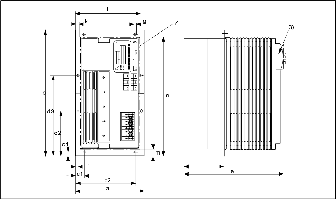
FIG 4-8 Abmessungen 8215 - 8218: Montage mit thermisch separiertem Leistungsteil
