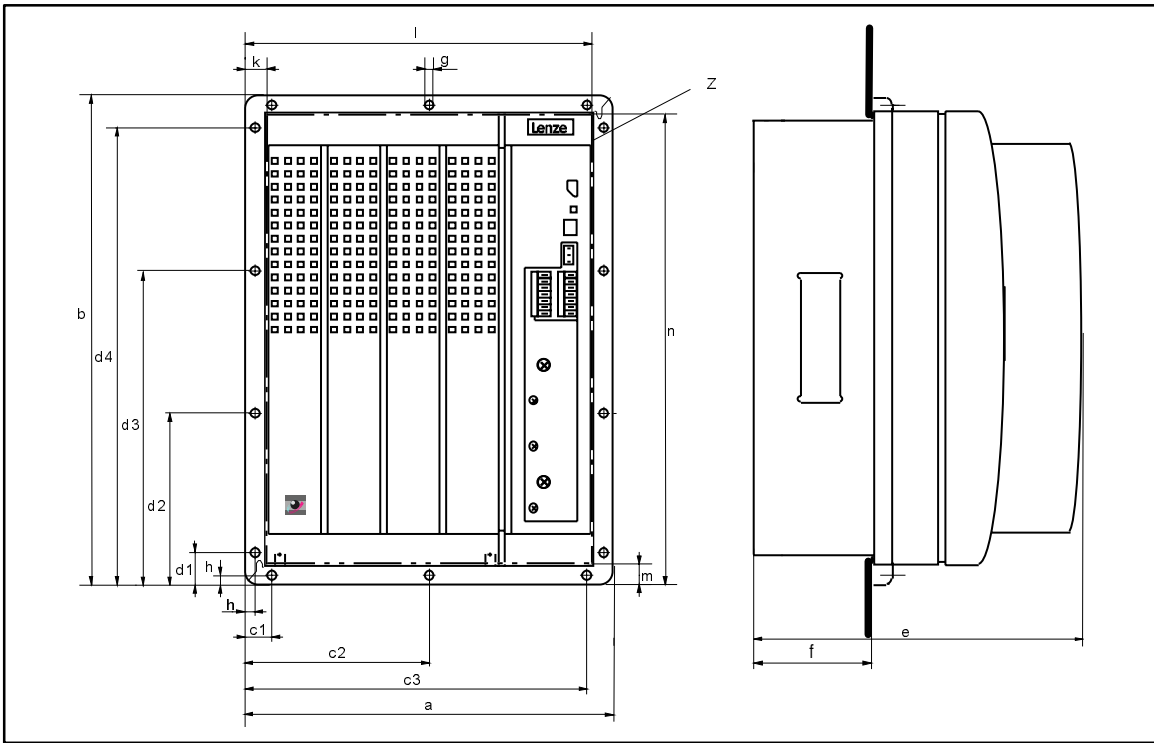
FIG 4-9 Abmessungen 8221 - 8227: Montage mit thermisch separiertem Leistungsteil
