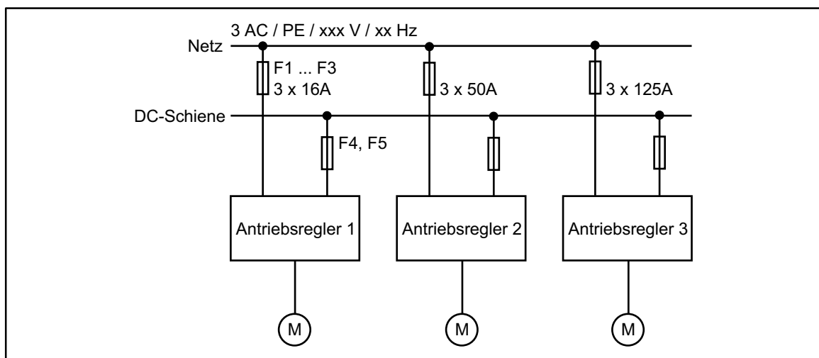
FIG 10-1 Beispiel zur Bemessung des Leitungsquerschnitts der DC-Schiene
