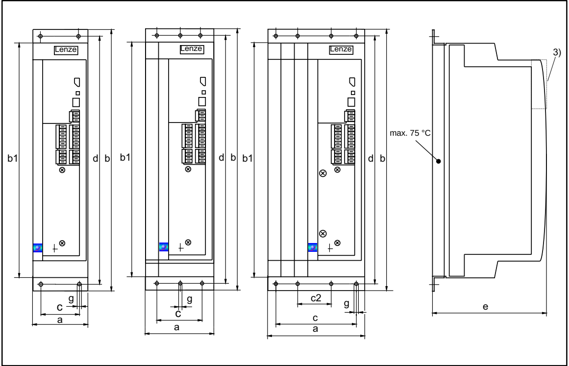
FIG 4-14 Abmessungen 824X-C-V003: Montage im Schaltschrank
