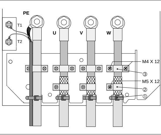
FIG 4-17 Vorschlag für Motoranschluß bei 822X
