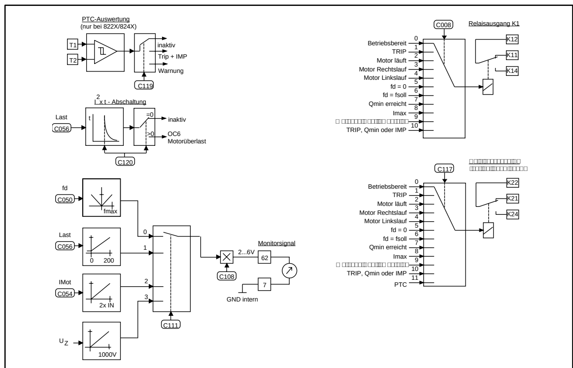
FIG 16-7 Signalfluß 821X/822X/824X: Überwachungen
