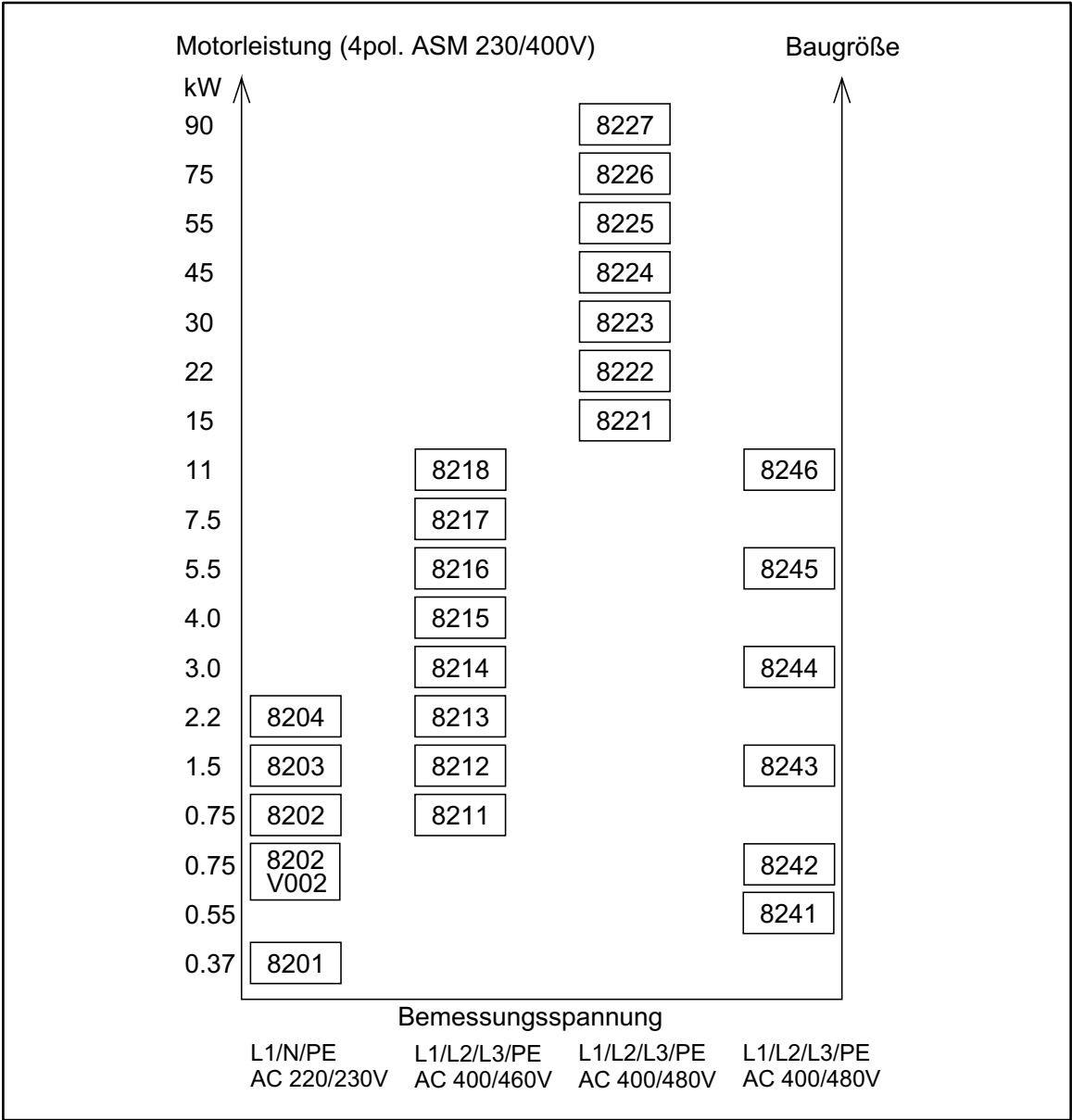
FIG 3-1 Typenübersicht
