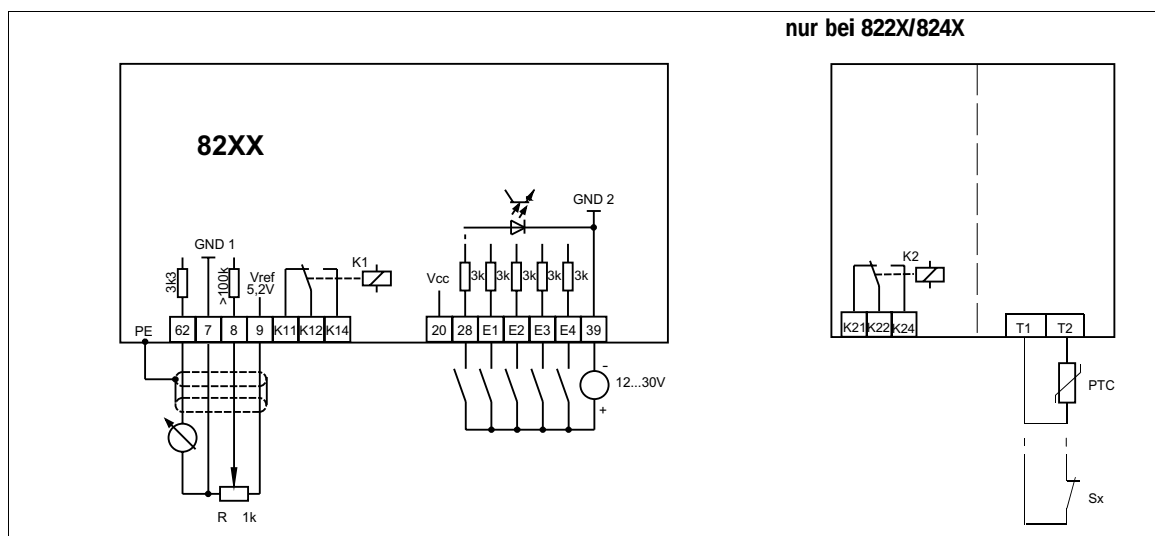
FIG 4-25 Steueranschlüsse: Versorgung mit externer Steuerspannung (+12 V ... +30 V)
