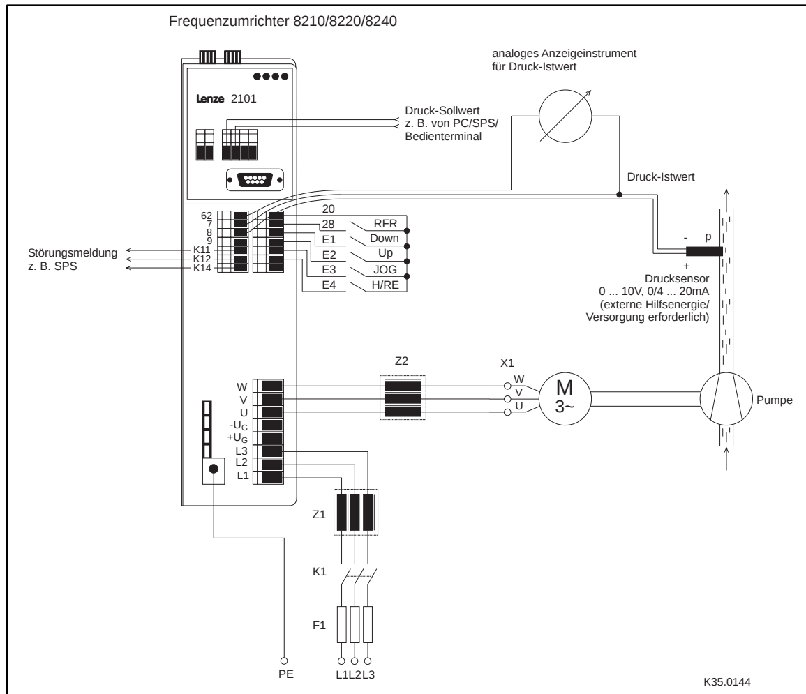
FIG 5-2 Einsatz einer Pumpe mit Druckregelung
