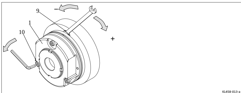
Abb. 5 Luftspalt nachstellen
