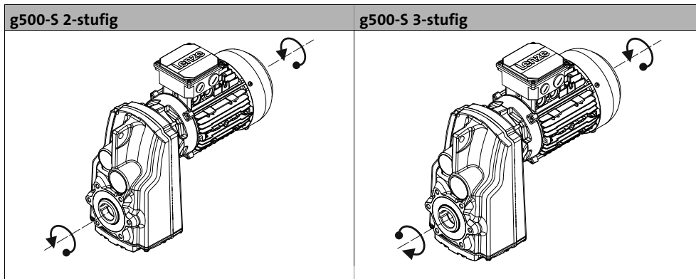
Abb. 2 Drehrichtung Antriebswelle (hier mit Drehstrommotor)
