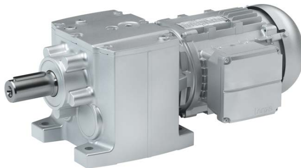
Getriebe g500-H450 mit Drehstrommotor m550-U80/M4
