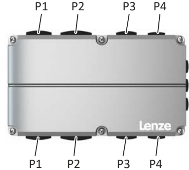
Klemmenkasten L
