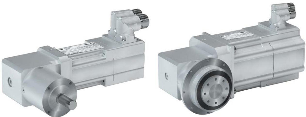
Kegelrad-Planetengetriebe g700-PB44 mit Servo-Synchronmotor MCS06 Kegelrad-Planetengetriebe g780-B130 mit Servo-Synchronmotor MCS12
