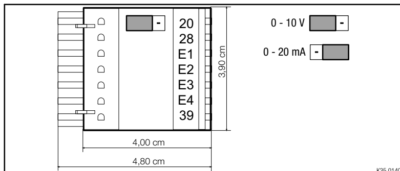
FIG 3-1 Abmessungen Analoges Anschaltmodul
