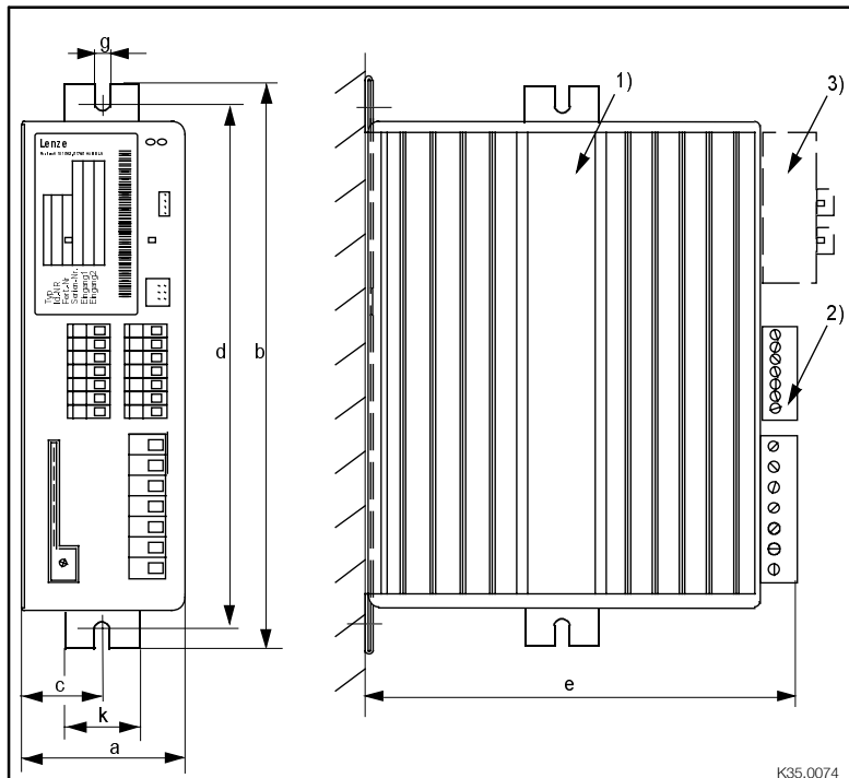
FIG 4-1 Abmessungen 8211 - 8214: Standardmontage
