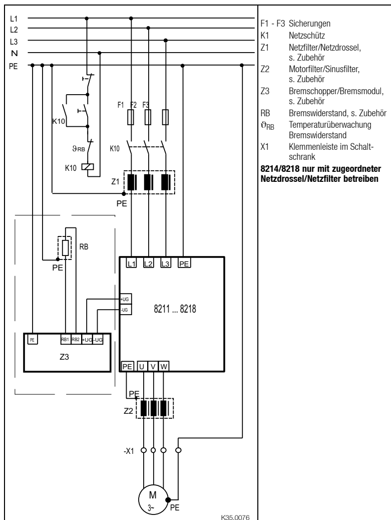
FIG 4-5 Leistungsanschlüsse 821X
