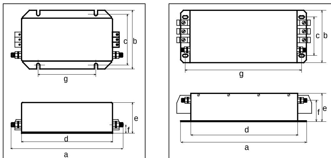
Bauform A
