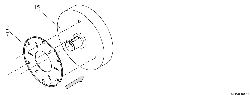
Abb. 6 Montage Reibblech
