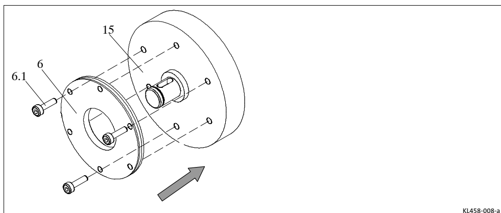
Abb. 7 Flanschmontage
