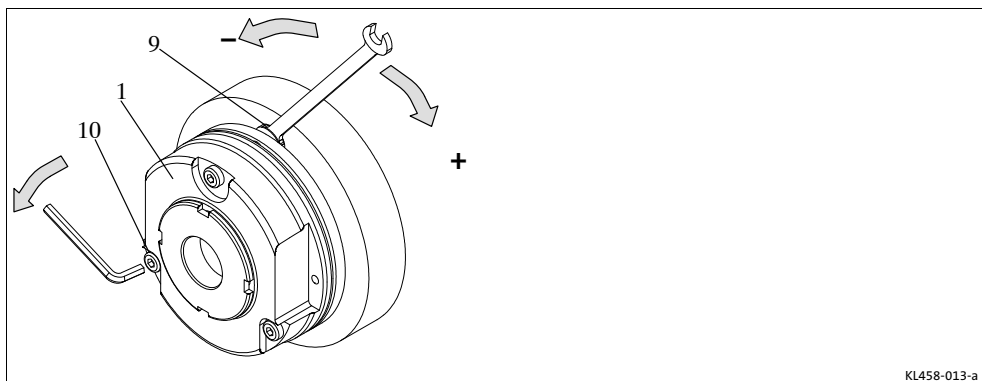
Abb. 5 Luftspalt nachstellen
