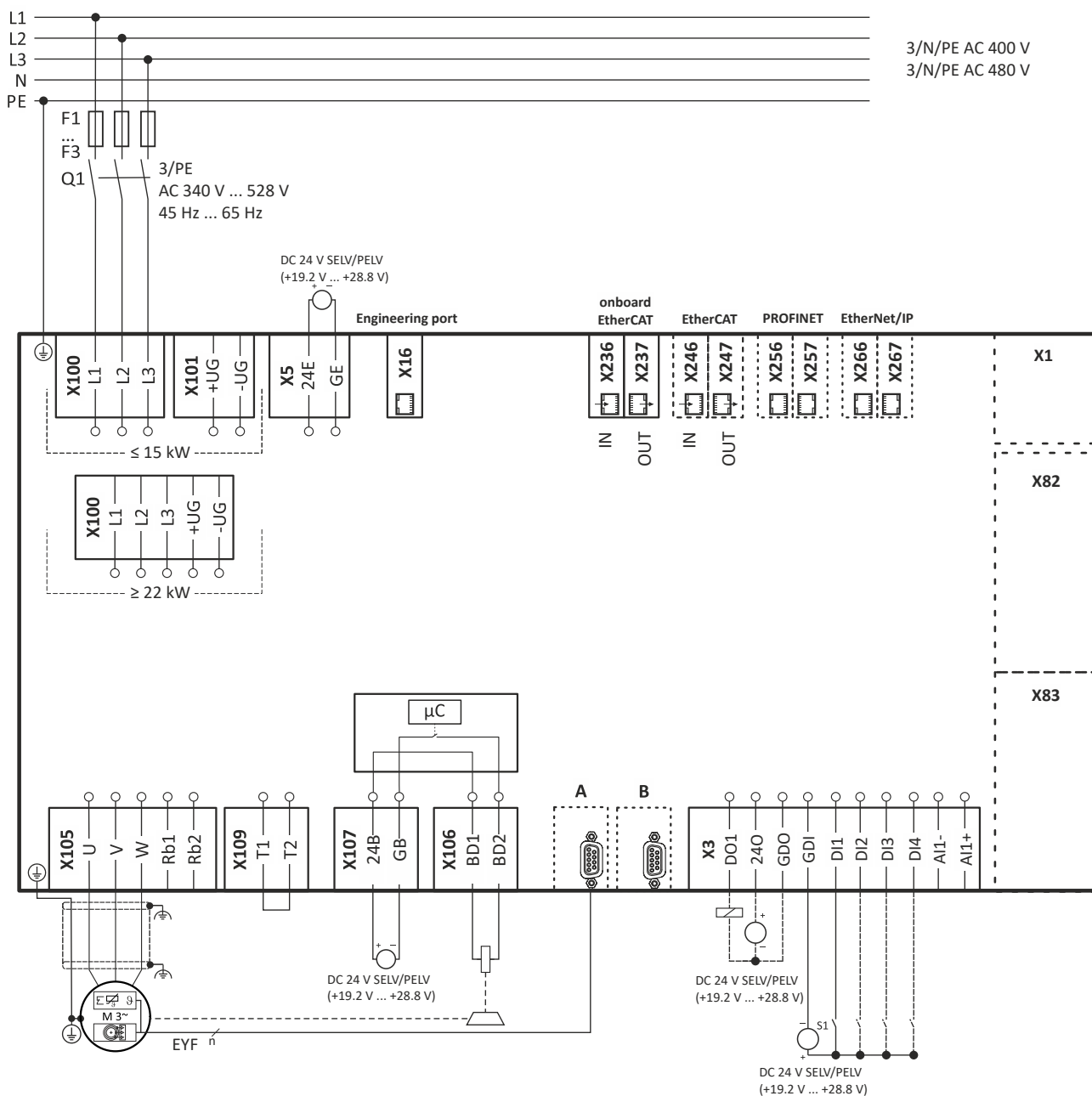
Fig. 4: Wiring example
