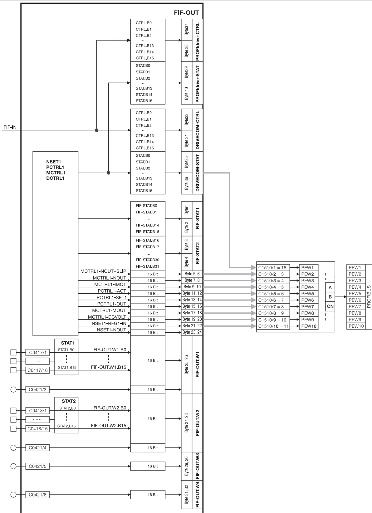
Abb. 7-2 Freie Konfiguration der 10 Prozess-Eingangswörter des PROFIBUS
