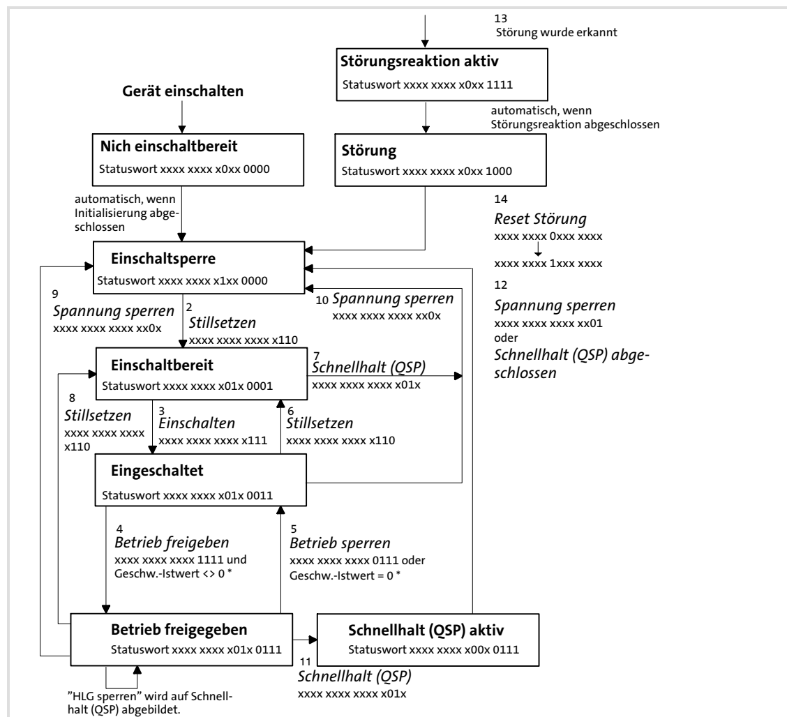
Abb. 7-3 Zustandsdiagramm DRIVECOM-Gerätesteuerung
