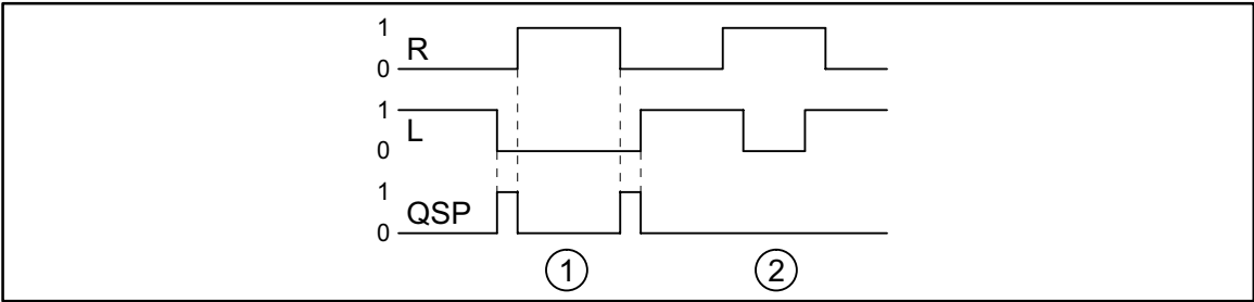
FIG 5-3 Drehrichtungsvorgabe
