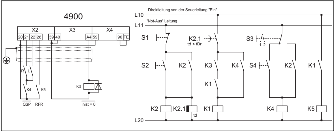
FIG 15-10 Anschluß der Signalelektronik für Tippbetrieb über Taster S4
