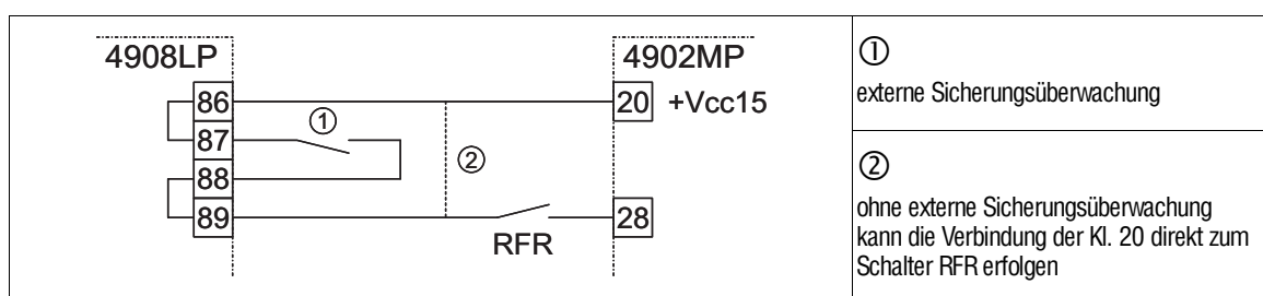
FIG 4-13 4808...4809 und 4908...4909
