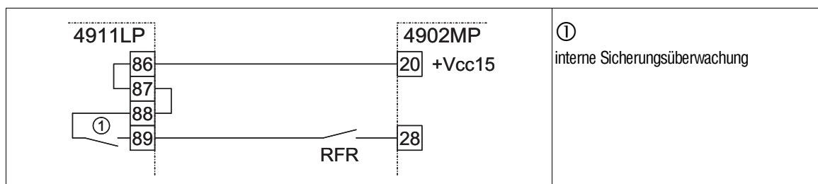
FIG 4-14 4811...4813 und 4911...4913
