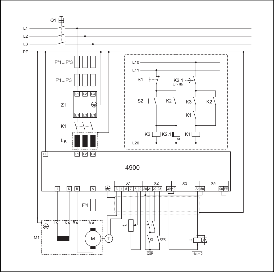
FIG 5-1 Schaltungsausschnitt: Drehzahlregelung mit Tacho
