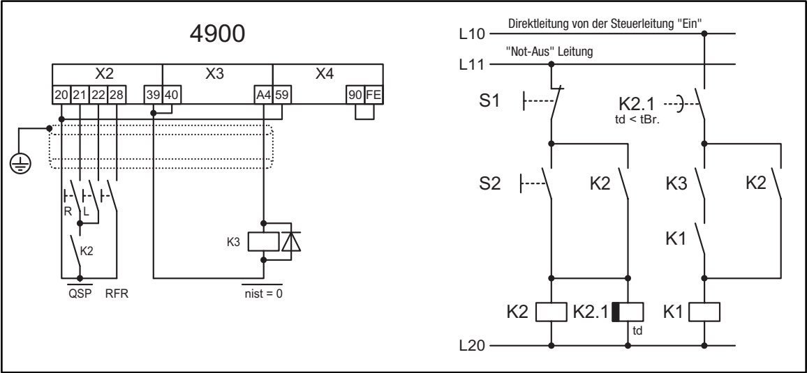
FIG 15-11 Beispiel für schnellstmögliches Abschalten im Wechselrichterbetrieb AP_ABSCH
