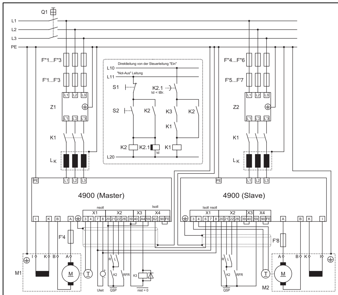
FIG 15-4 Anschlußschaltbild Stromverhältnisregelung
