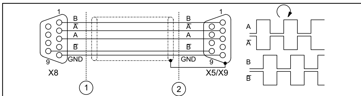
FIG 4-18 Leitfrequenzvorgabe für Folgeantrieb ② über LF-Ausgang (Leitantrieb ①)
