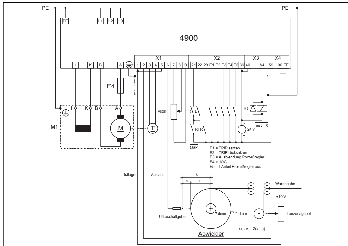
FIG 15-5 Signalflußplan Tänzerlageregelung an einem Abwickler
