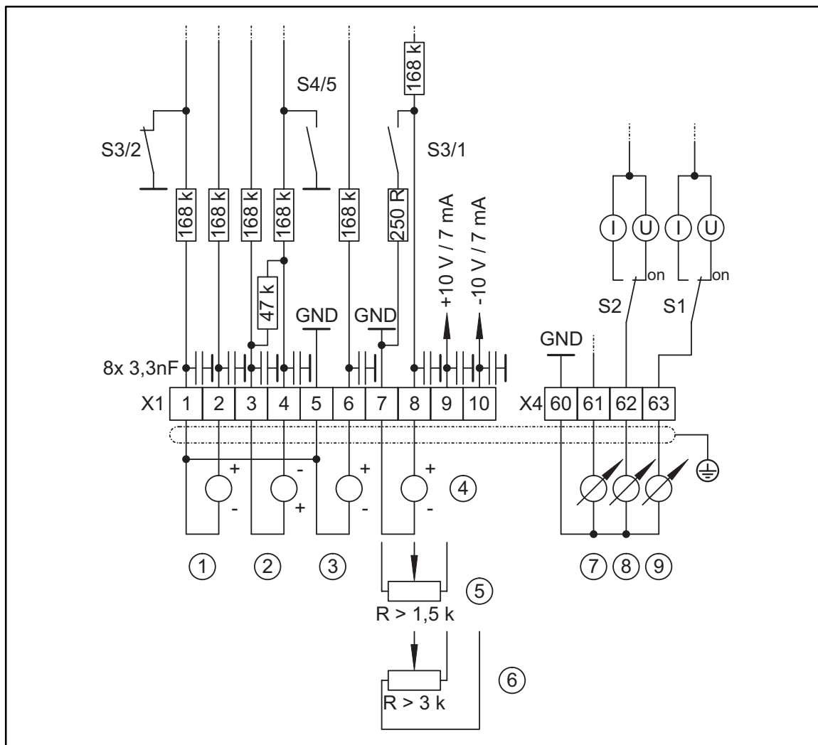
FIG 4-10 Analoge Ein- und Ausgänge
