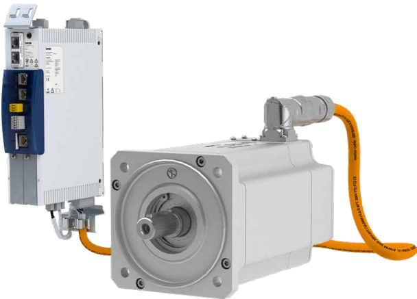
Rad s tehnologijom jednog kabela (OCT)
