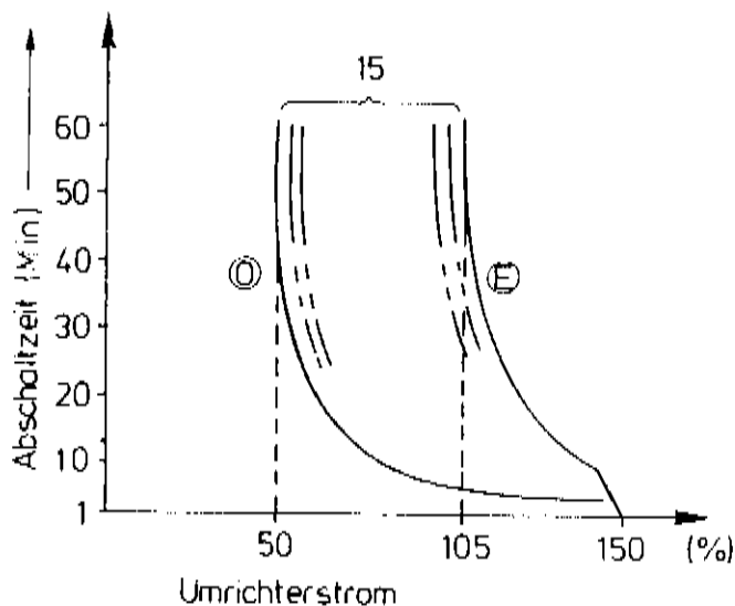
Kennlinie 1
