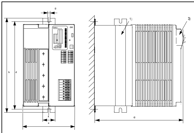
FIG 4-2 Abmessungen 8215 - 8218: Standardmontage
