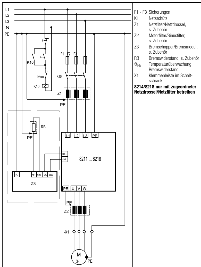
FIG 4-6 Leistungsanschlüsse 821X
