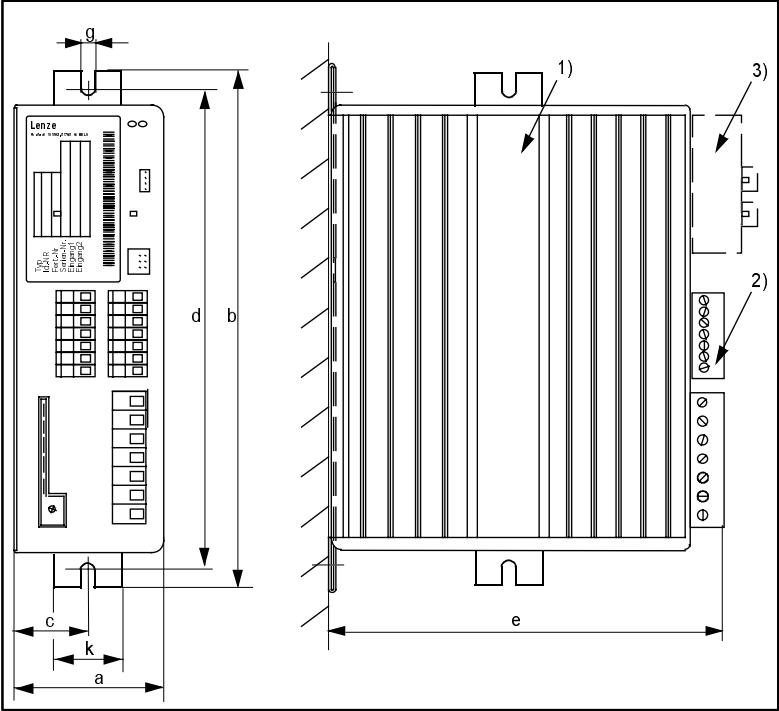
FIG 4-1 Abmessungen 8211 - 8214: Standardmontage 1) bei seitlicher Montage Befestigungsschiene hier einschleiben 2) Montagefreiraum für Anschlußkabel berücksichtigen 3) mit aufsteckbarem Feldbus- oder I/O-Modul: Montagetiefe und benötigten Montagefreiraum für Anschlußkabel berücksichtigen
