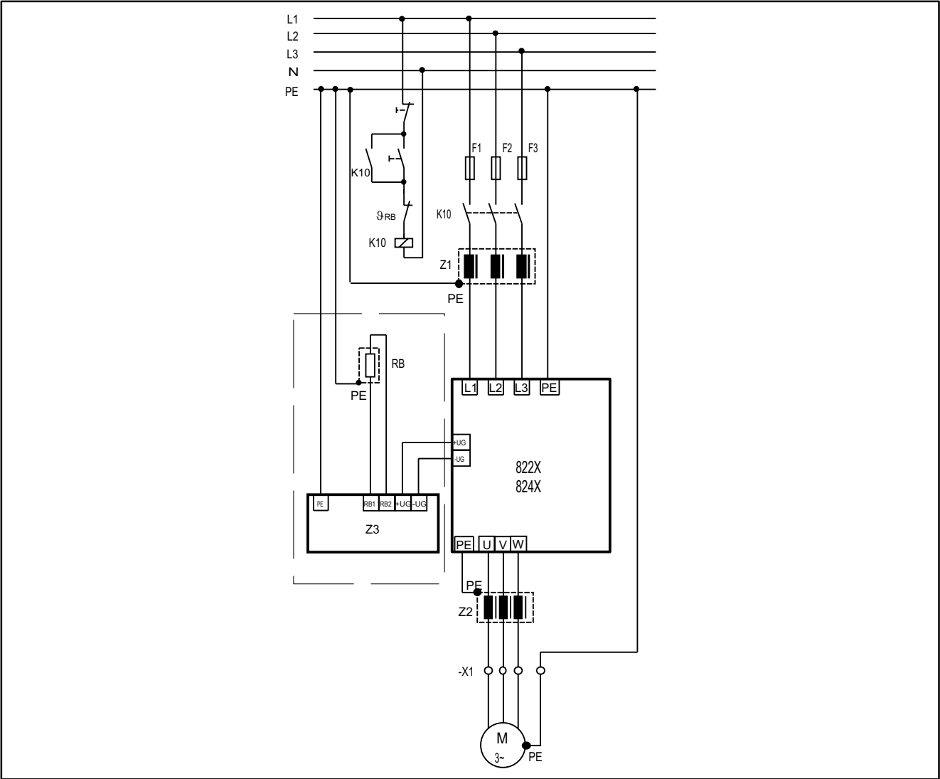
Abb. 4-6 Leistungsanschlüsse 822X/824X
