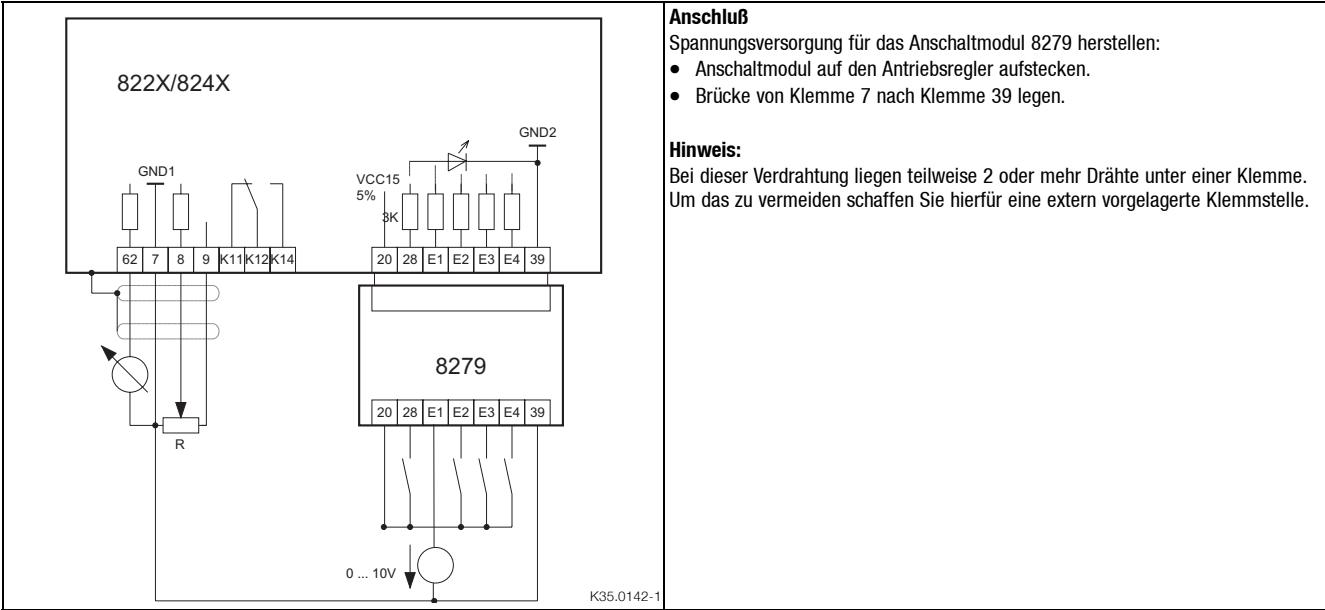
Abb. 4-10 Steueranschlüsse: Versorgung mit interner Steuerspannung
