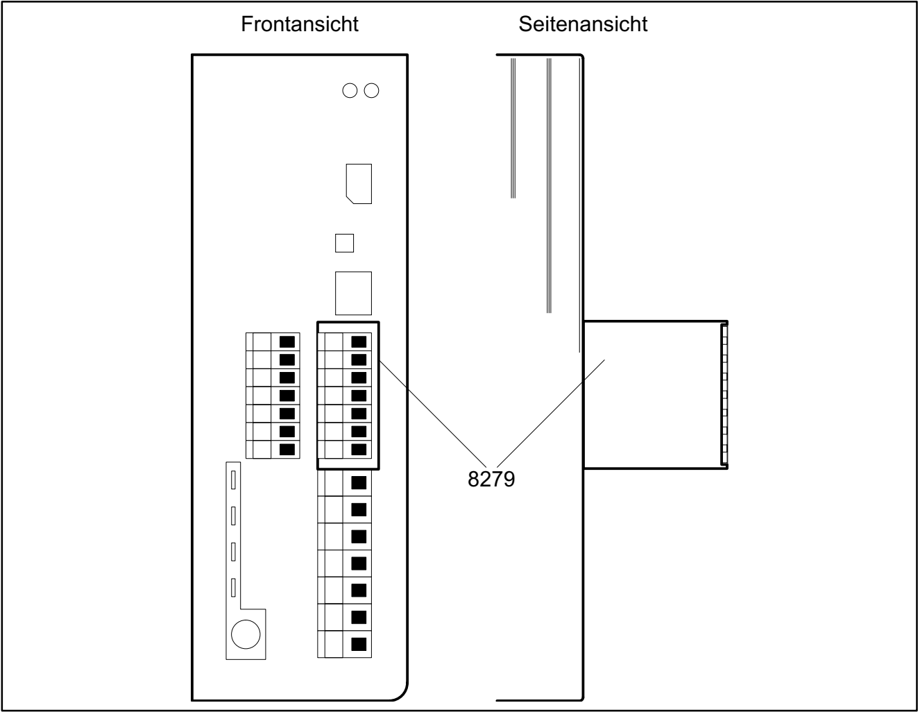
Abb. 4-2 Analoges Anschaltmodul am Antriebsregler montiert
