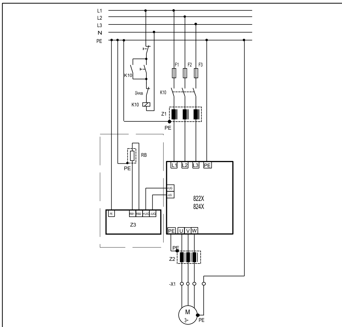
FIG 4-8 Leistungsanschlüsse 822X/824X
