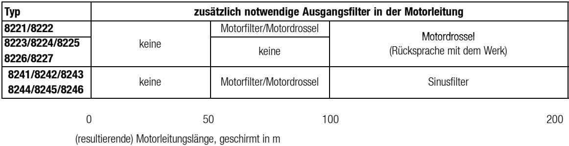
FIG 4-7 Zusätzlich notwendige Ausgangsfilter in der Motorleitung
