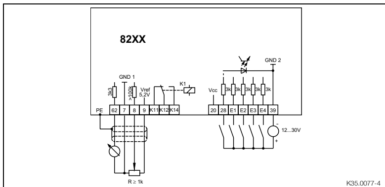
FIG 4-7 Steueranschlüsse: Versorgung mit externer Steuerspannung (+12 V ... +30 V) GND1 Bezugspunkt für interne Spannungen GND2 Bezugspunkt für externe Spannungen GND1 und GND2 sind geräteintern potentialgetrennt
