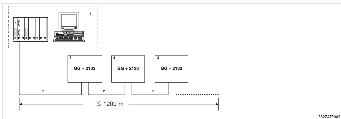
Abb. 5-2 Beispiel: PROFIBUS mit RS485-Verkabelung (ohne Repeater)
