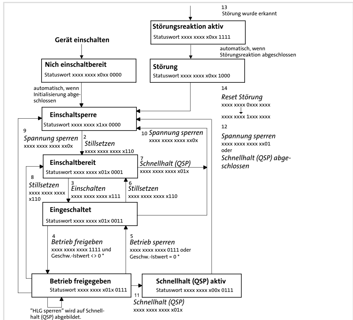
Abb. 7-10 Zustandsdiagramm DRIVECOM-Gerätesteuerung
