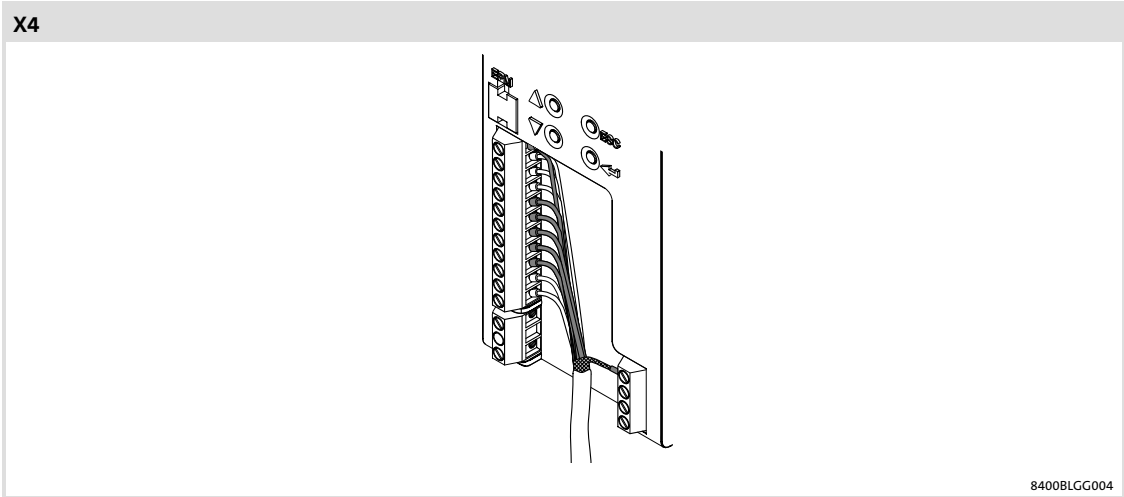
Fig.6-20 Cablaggio e schermatura degli ingressi digitali DO1 L'uscita digitale non è disponibile per dispositivi con codice E84AVBDxxxxSX0 (v. targhetta)
