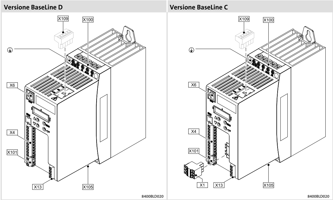
Fig.4-2 Versione BaseLine, dispositivi nel campo di potenza da 0.25 a 3 kW
