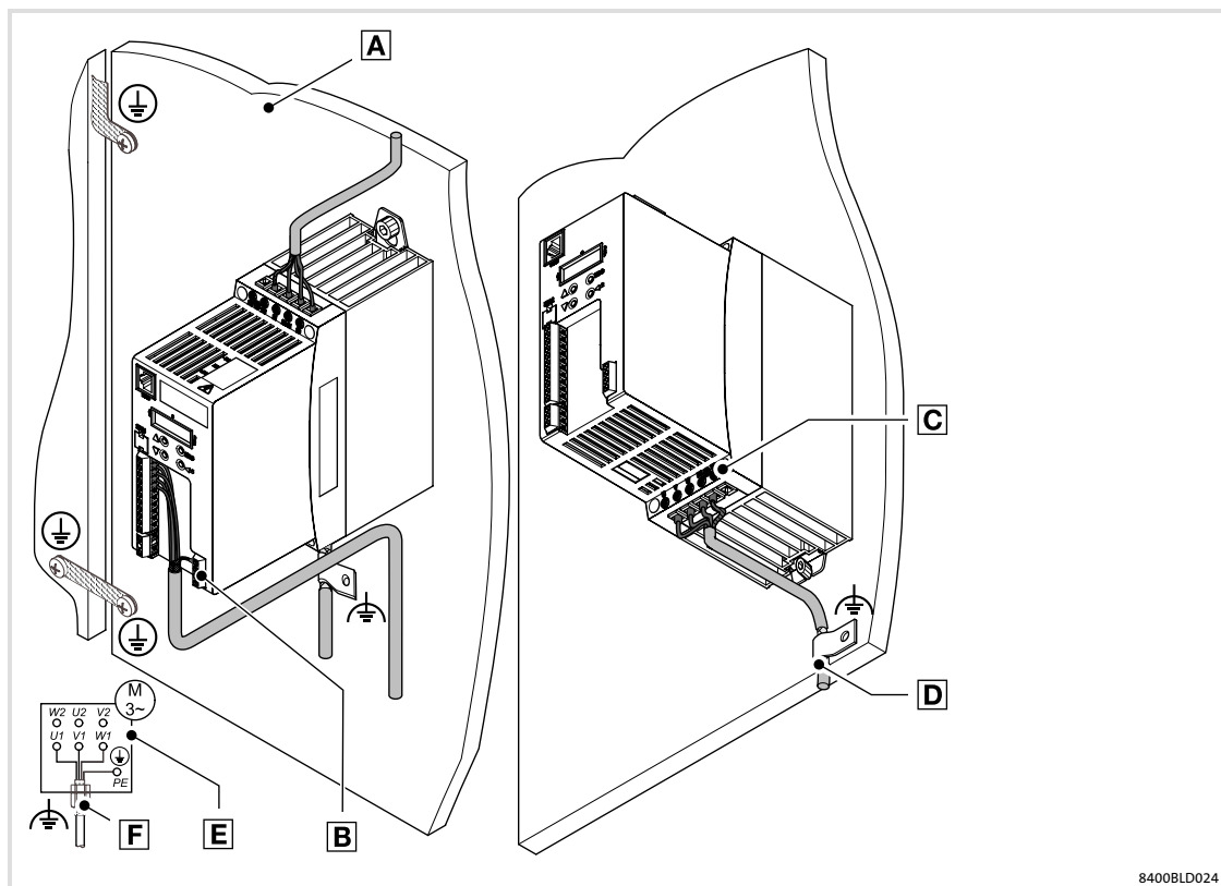
Fig.6-2 Cablaggio conforme EMC
