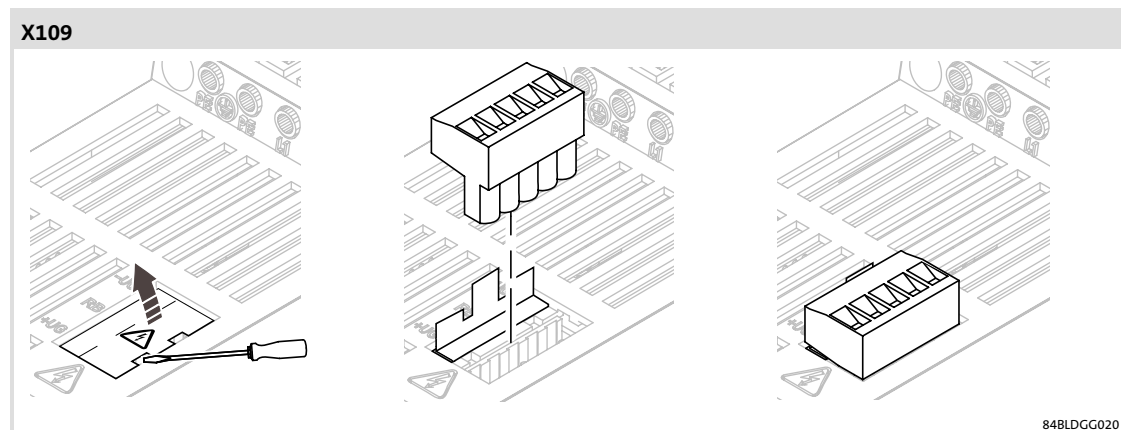
Fig.6-10 Inserimento della morsettiera X109
