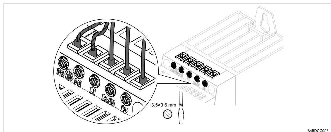
Fig.6-12 Collegamento lato rete del dispositivo alla terra di protezione
