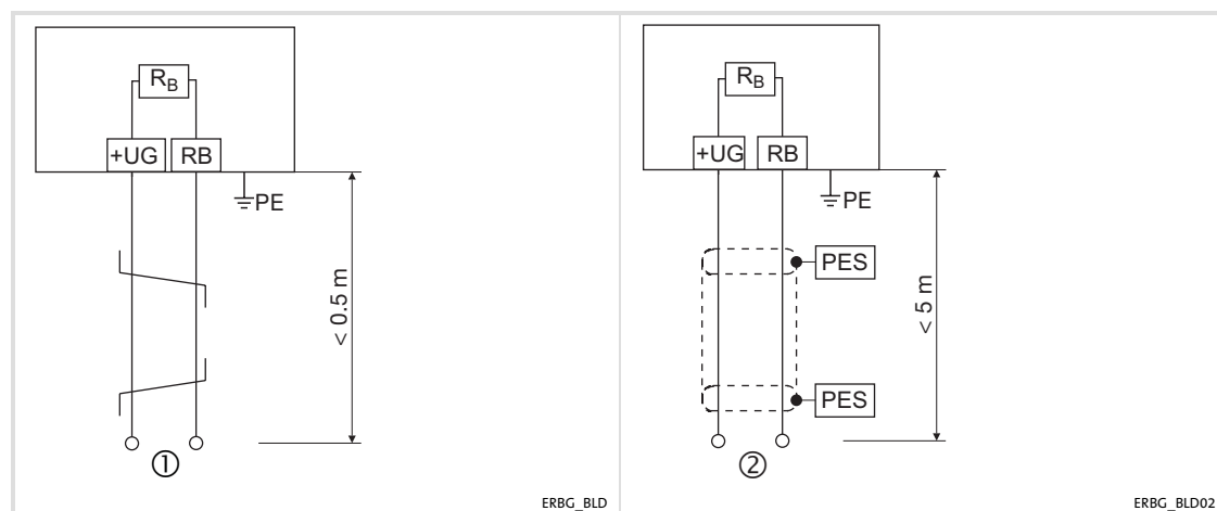
Fig.8-2 Cablaggio di una resistenza di frenatura sull'unità di controllo
