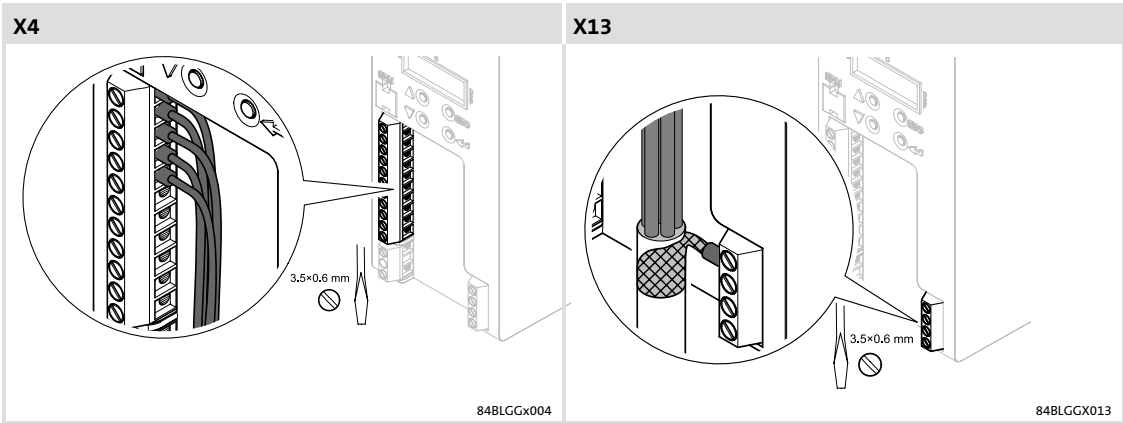
Fig.6-15 Schermare e collegare i cavi di controllo
