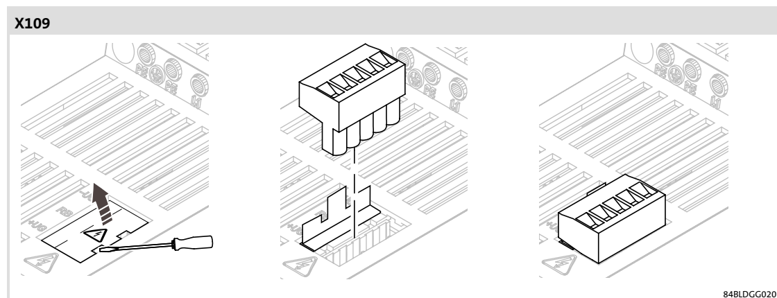
Fig.6-14 Inserimento della morsettiera X109
