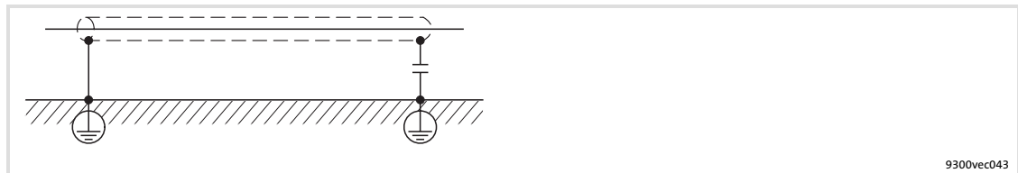
Fig.6-4 Schermatura di lunghi cavi di controllo analogici
