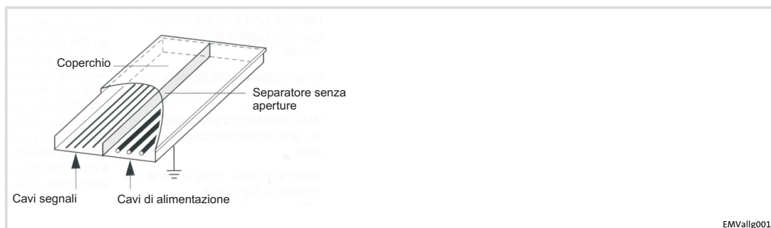
Fig.6-6 Cavi posati in canalina con parete di separazione
