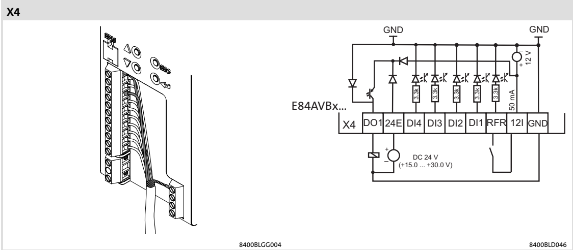
Fig.6-19 Collegamento alla tensione di alimentazione esterna
