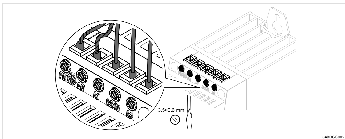
Fig.6-9 Collegamento lato rete del dispositivo alla terra di protezione
