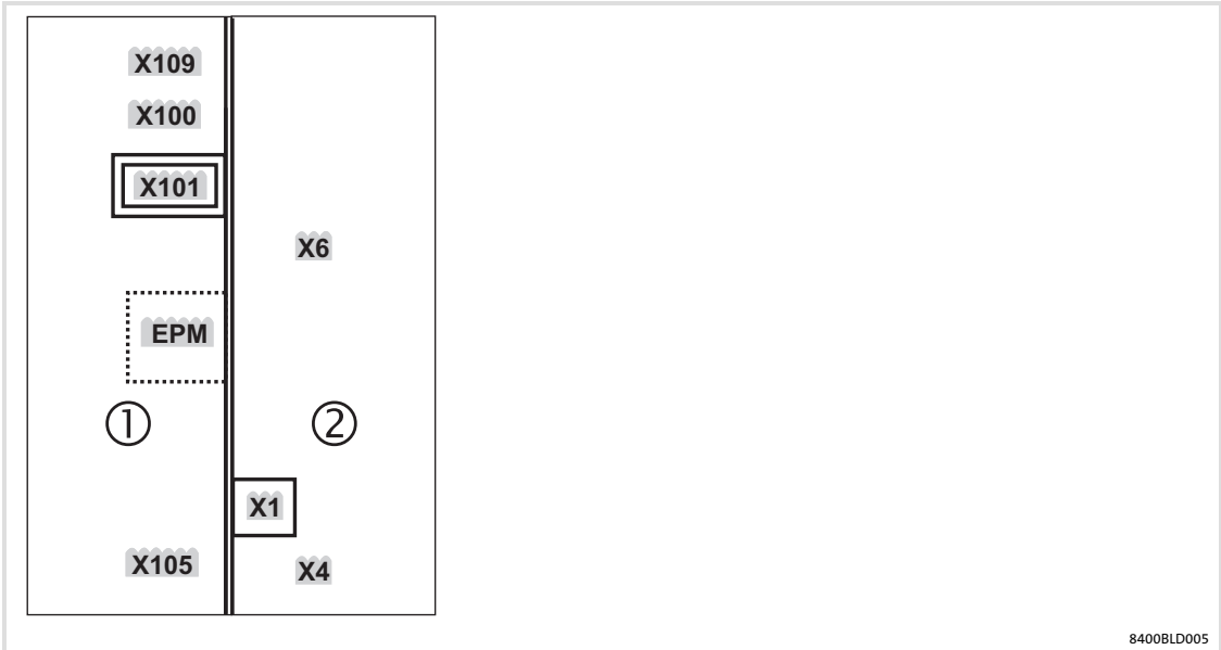
Fig.6-1 Separazione del potenziale tra i morsetti di potenza, i morsetti di controllo e la carcassa
