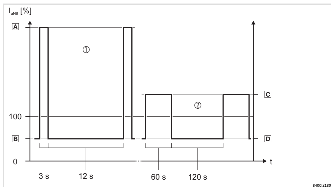
Fig.4-1 Capacità di sovracorrente nel funzionamento a 230/400 V a 45° C
