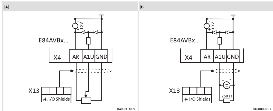
Fig.6-18 Esempi di collegamento per l'ingresso analogico
