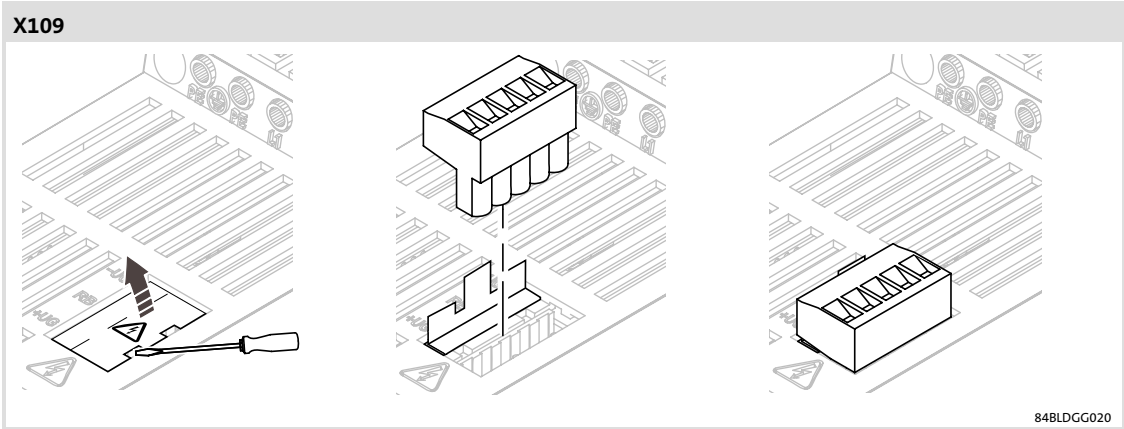
Fig.6-13 Inserimento della morsettiera X109
