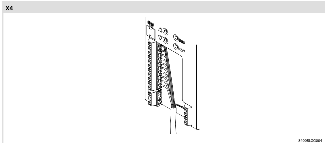
Fig.6-17 Cablaggio e schermatura dell'ingresso analogico
