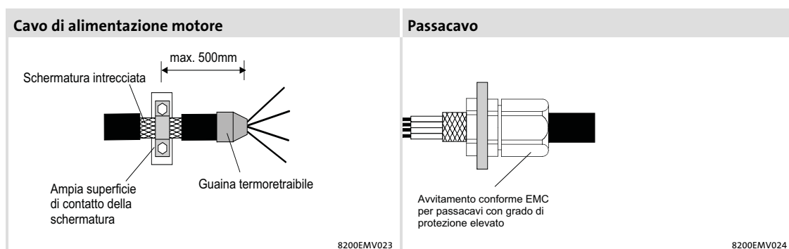
Fig.6-3 Schermatura del cavo motore
