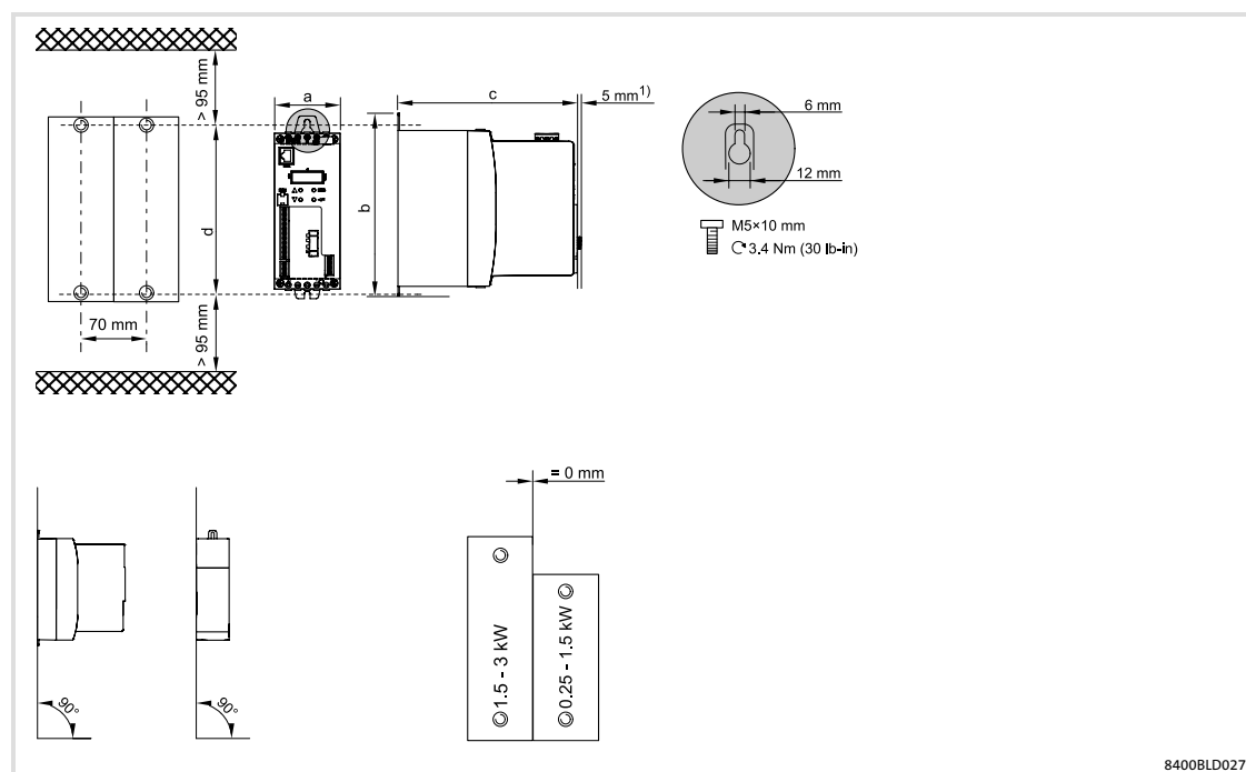
Fig.5-1 Montaggio ad incasso (standard)
