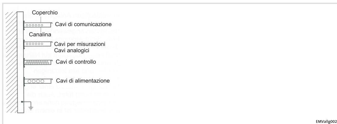
Fig.6-7 Cavi posati in canaline separate
