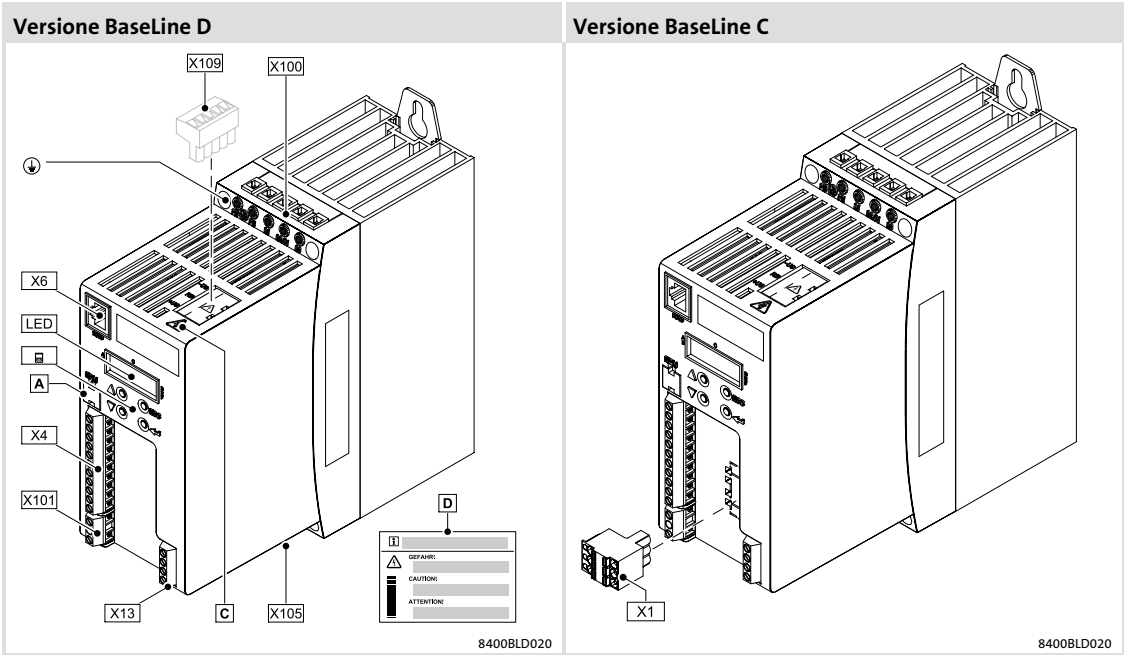
Fig.3-1 Versione BaseLine, dispositivi nel campo di potenza da 0.25 a 3 kW
