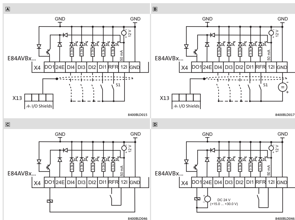
Fig.6-21 Esempi di collegamento per gli ingressi digitali
