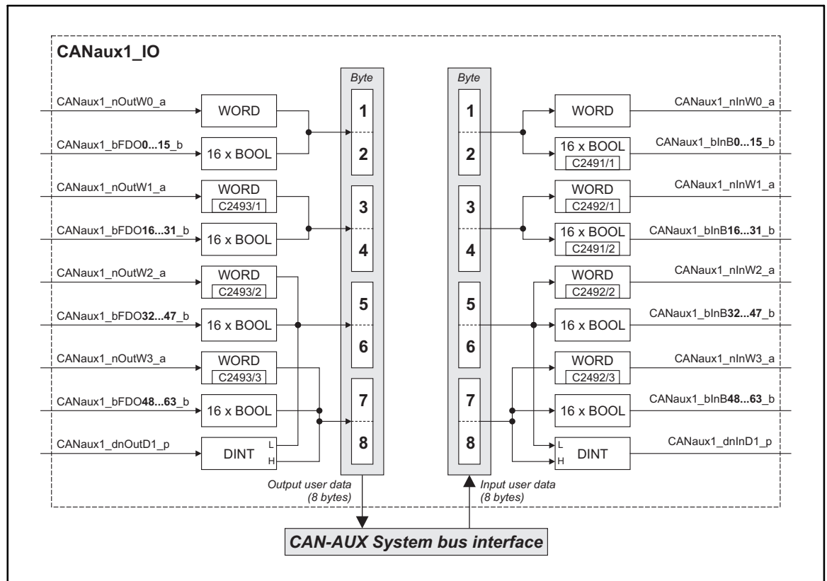
CANaux1_IOsystem block
