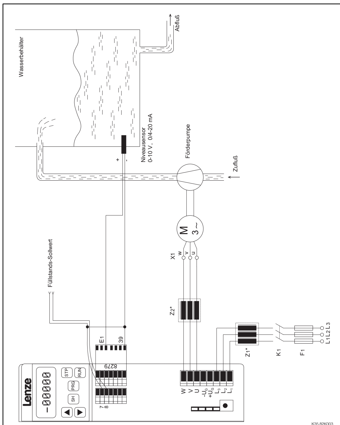
FIG 5-3 Einsatz einer Pumpe mit Niveauregelung
