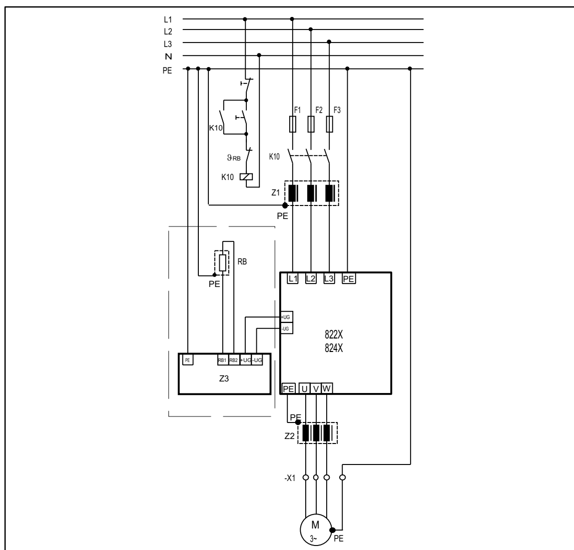
FIG 4-6 Leistungsanschlüsse 822X/824X
