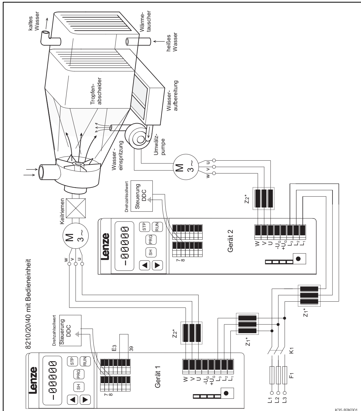
FIG 5-1 Anwendungsbeispiel einer Klimaanlage
