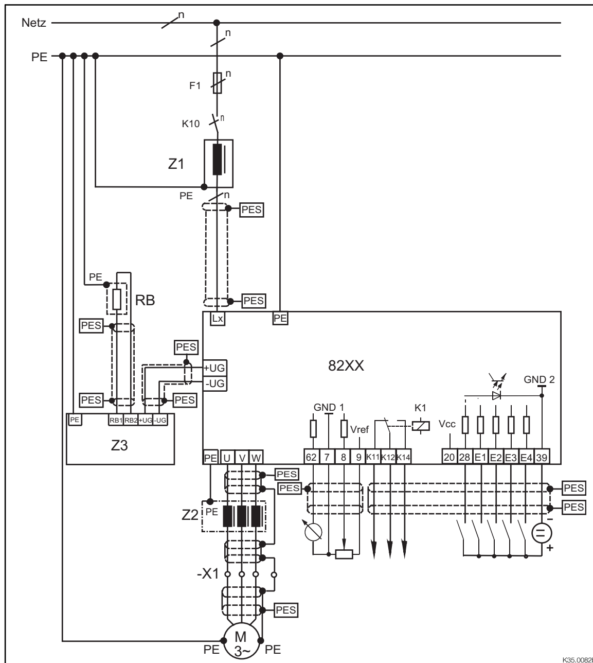
FIG 4-12 Beispiel für eine EMV-gerechte Verdrahtung
