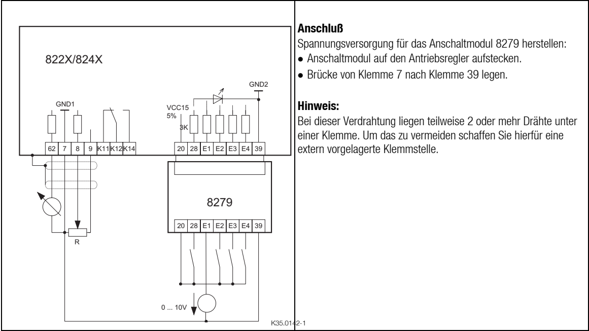
FIG 4-10 Steueranschlüsse: Versorgung mit interner Steuerspannung
