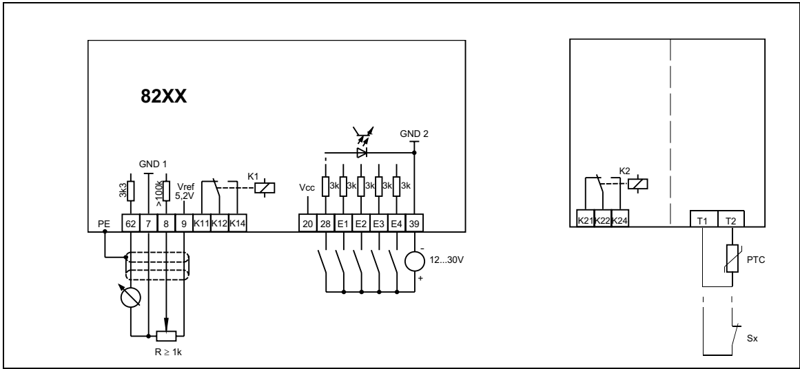
FIG 4-9 Steueranschlüsse: Versorgung mit externer Steuerspannung (+12 V ... +30 V)
