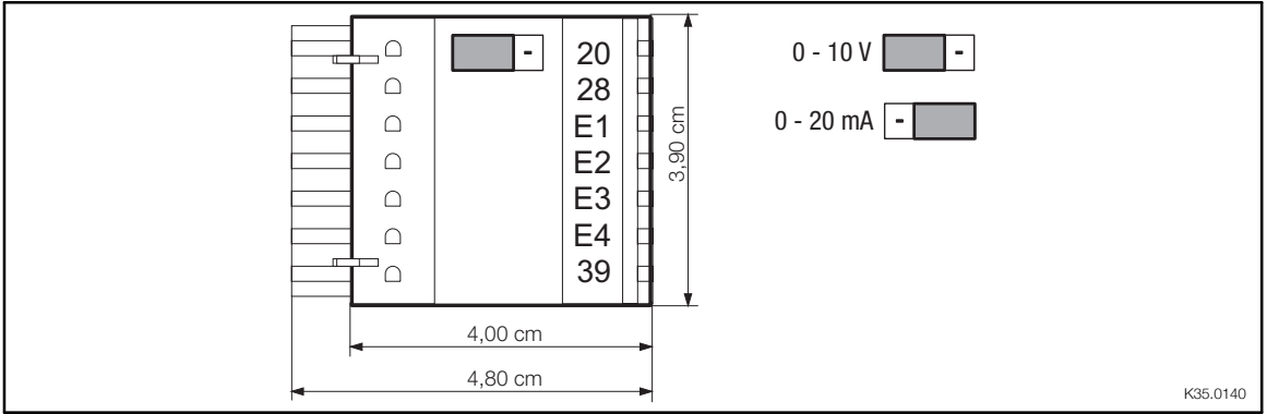
FIG 3-1 Abmessungen Analoges Anschaltmodul
