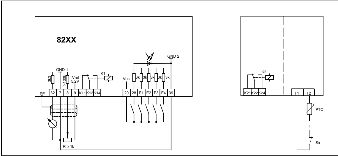
FIG 4-8 Steueranschlüsse: Versorgung mit interner Steuerspannung
