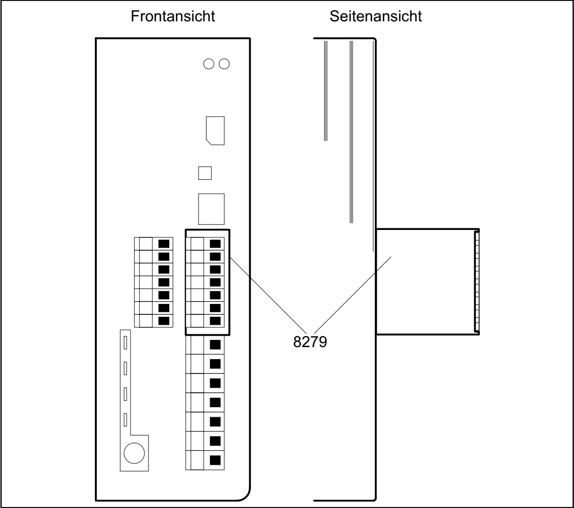
FIG 4-2 Analoges Anschaltmodul am Antriebsregler montiert
