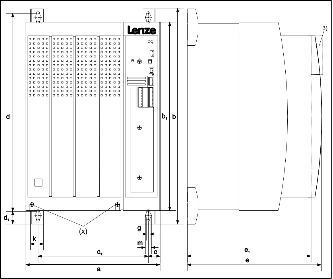
FIG 4-1 Abmessungen Standardmontage
