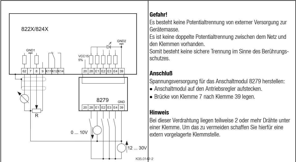
FIG 4-11 Steueranschlüsse: Versorgung mit externer Steuerspannung (+12 ... +30 V)
