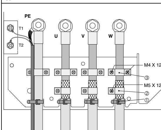
FIG 4-4 Vorschlag für Motoranschluß bei 822X
