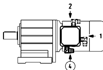
端子盒在位置5
