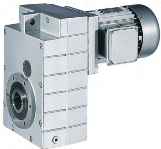
小侧隙减速电机 GFL07-2M HCR 100-32
