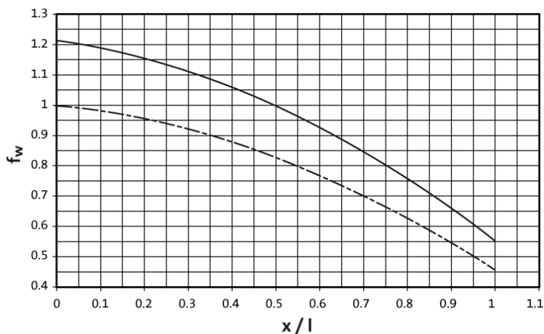
Lastangriffsbeiwert f_w an der Abtriebswelle
