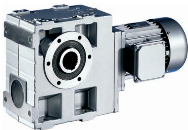
Kegelstirnradgetriebemotor GSS07-2M HBR 100-32
